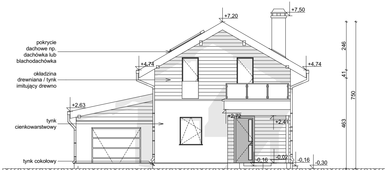
ELEWACJA FRONTOWA
