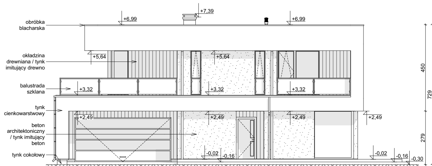
ELEWACJA FRONTOWA
