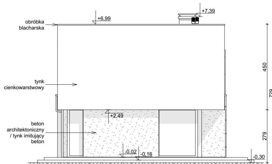
ELEWACJA BOCZNA
