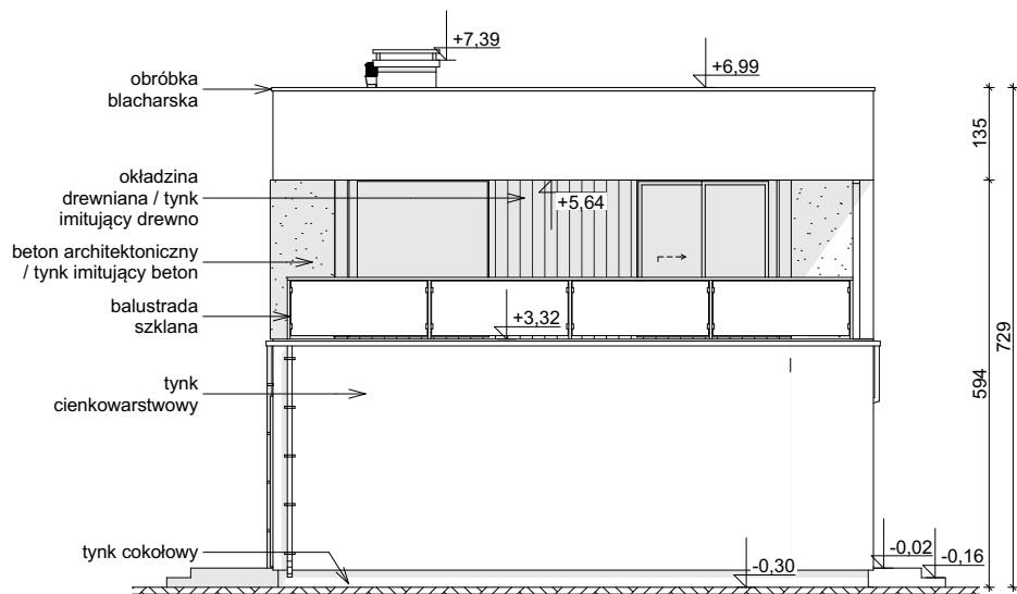
ELEWACJA BOCZNA
