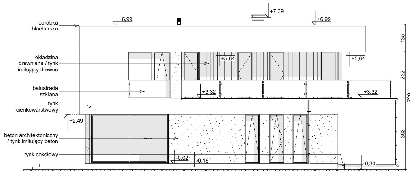
ELEWACJA OGRODOWA
