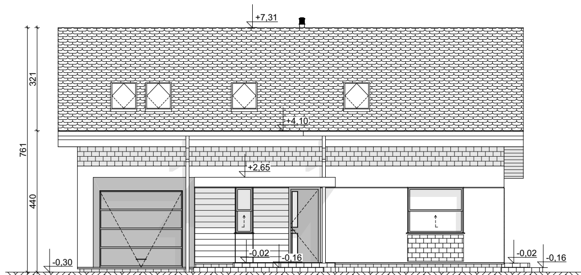
ELEWACJA FRONTOWA
