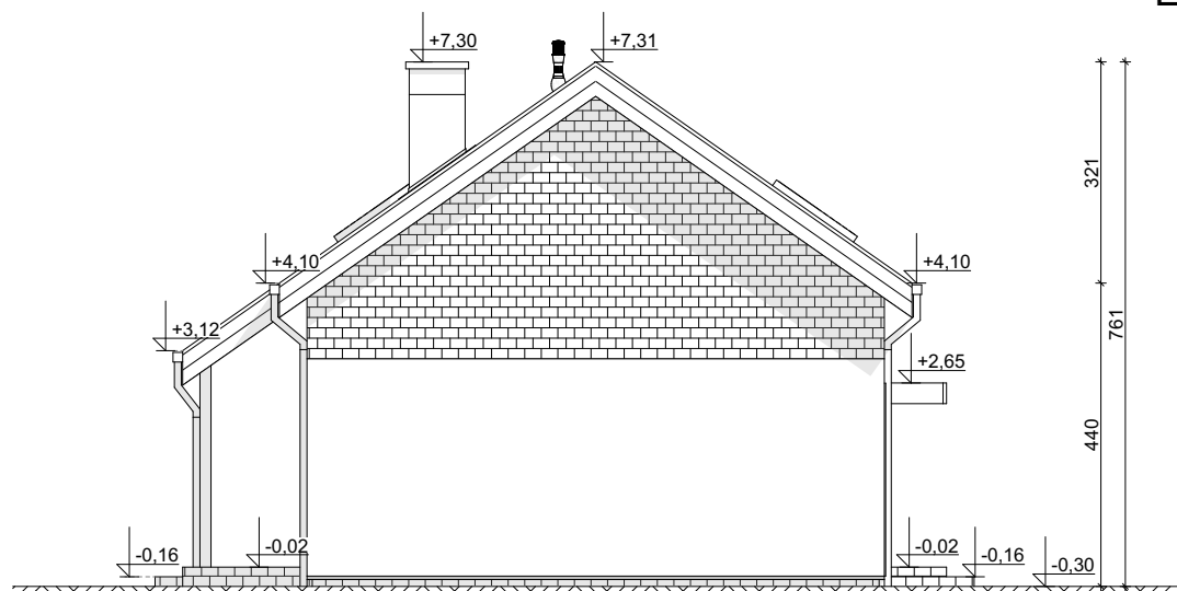
ELEWACJA BOCZNA
