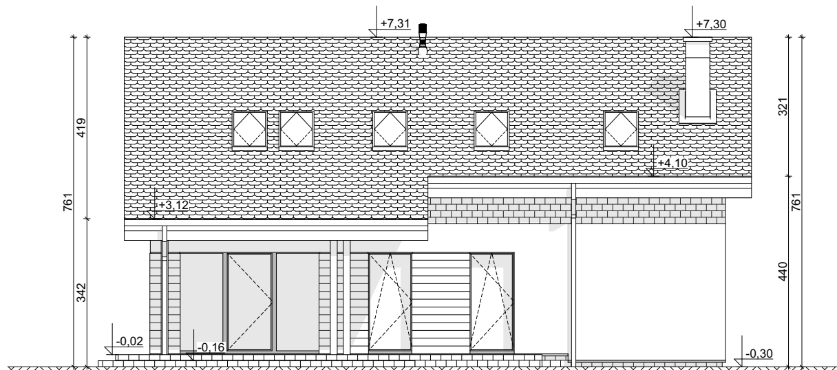
ELEVACJA OGRODOWA
