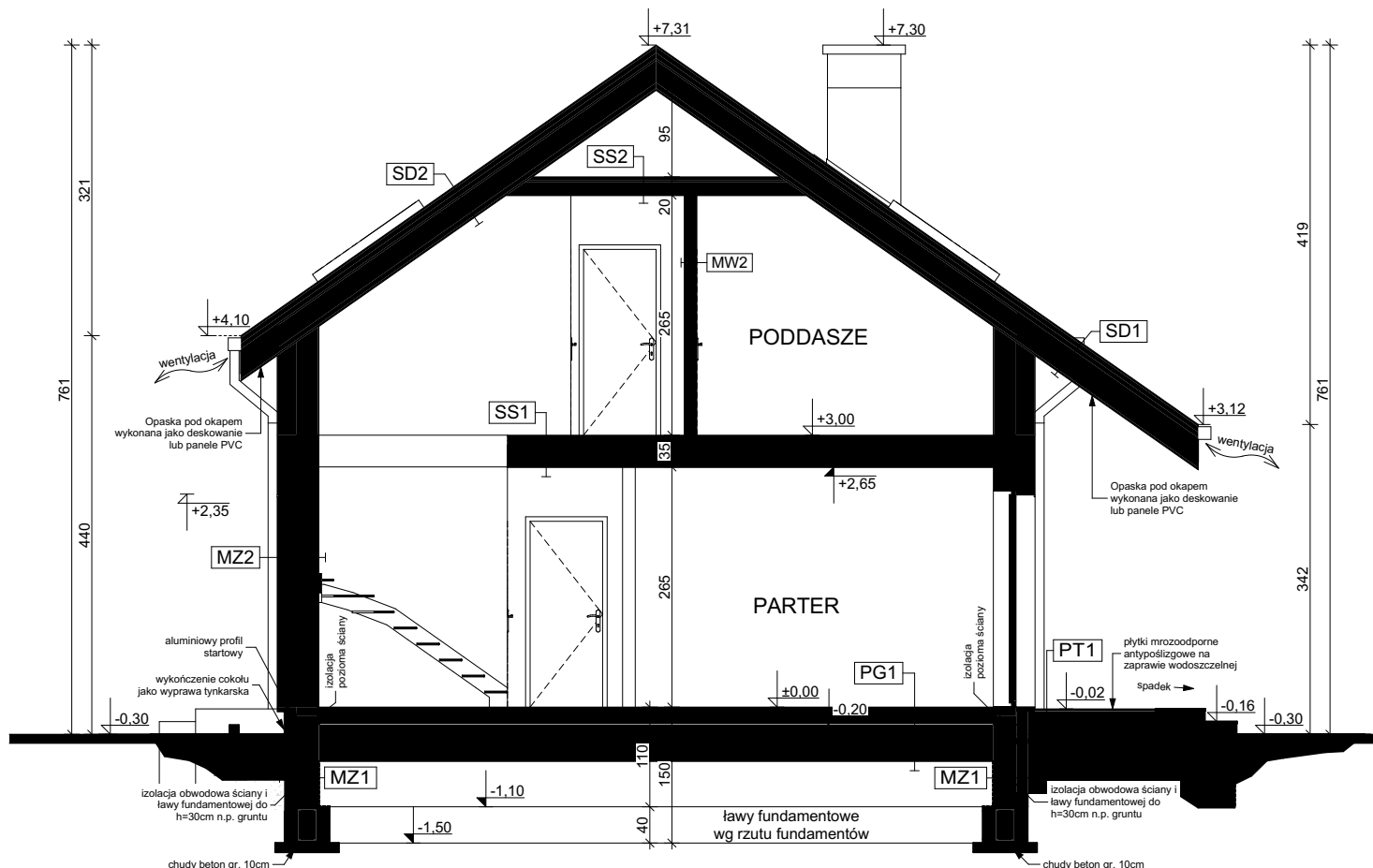
B-B PRZEKRÓJ
