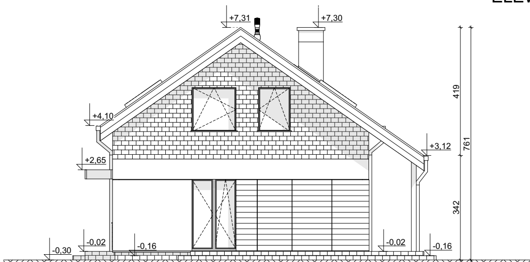
ELEVACJA BOCZNA
