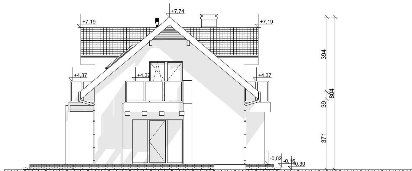
ELEVACJA BOCZNA
