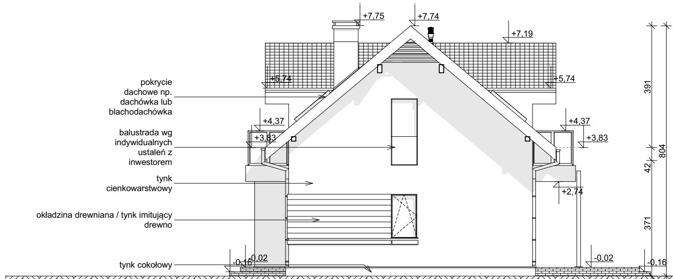
ELEVACJA BOCZNA
