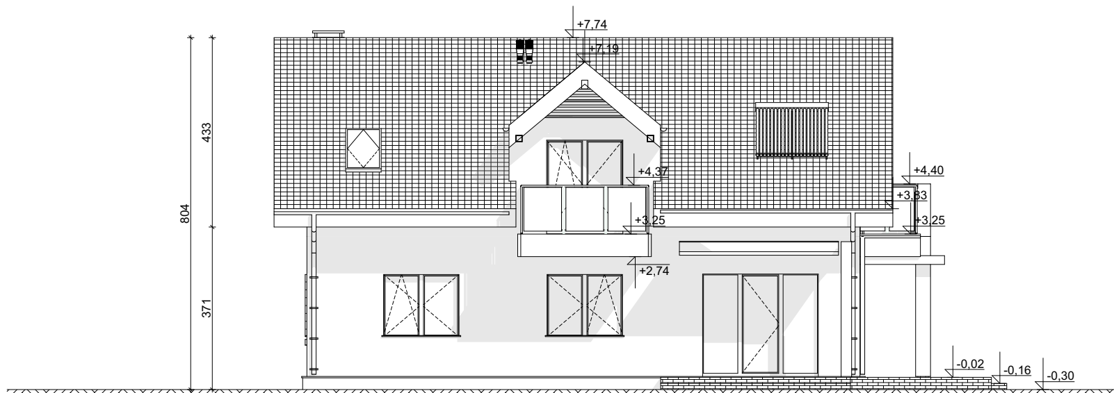
ELEVACJA OGRODOWA
