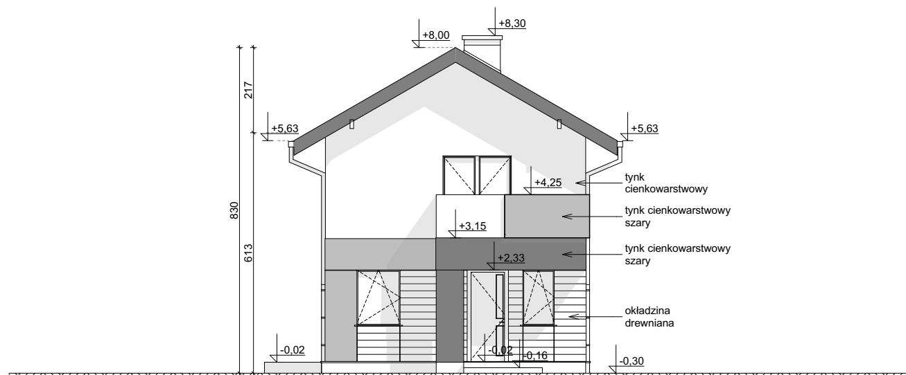
ELEWACJA FRONTOWA
