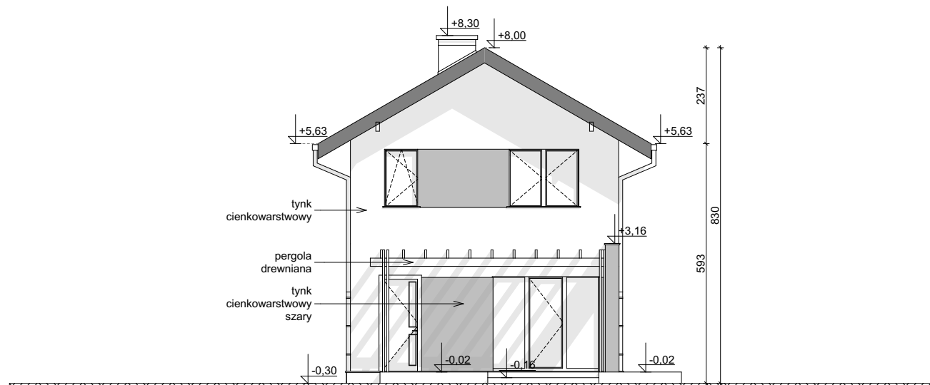
ELEWACJA OGRODOWA
