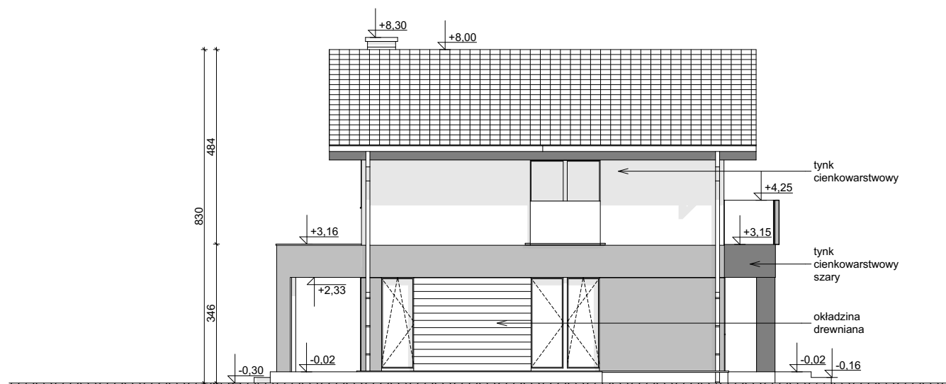
ELEWACJA BOCZNA
