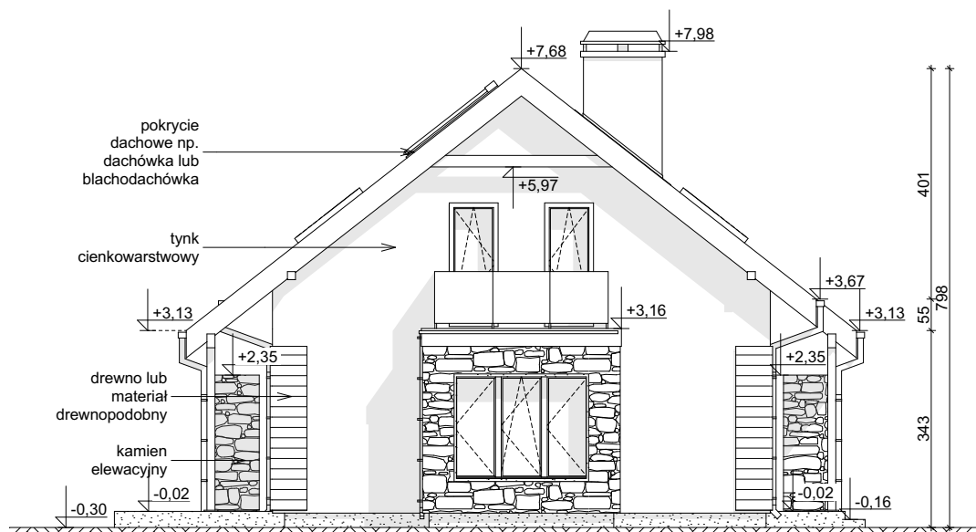
ELEWACJA BOCZNA
