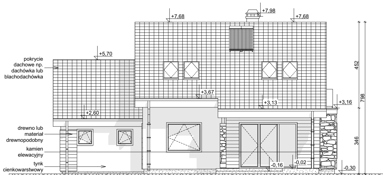
ELEWACJA OGRODOWA
