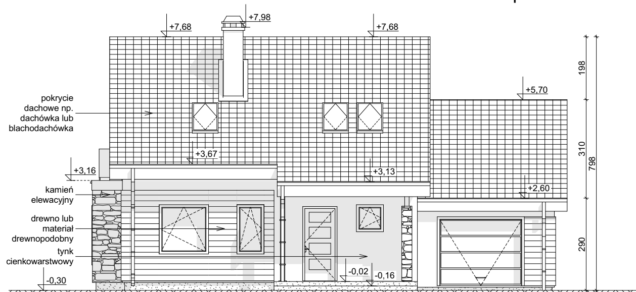
ELEWACJA FRONTOWA
