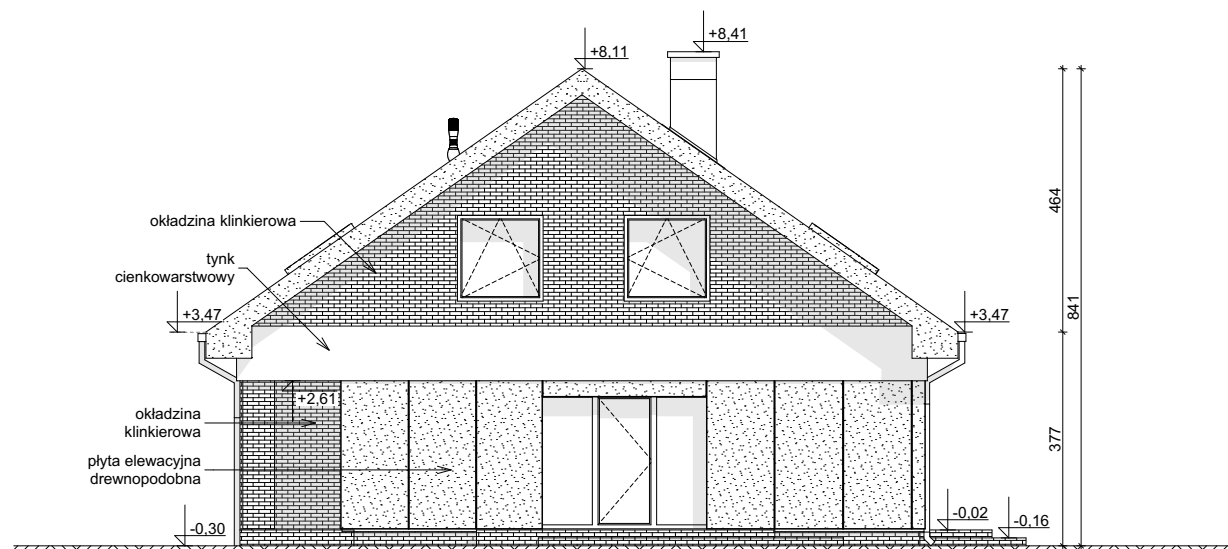
ELEWACJA BOCZNA
