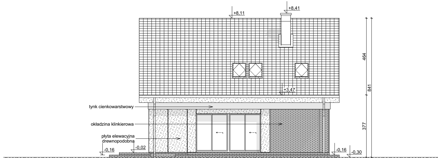
ELEWACJA OGRODOWA
