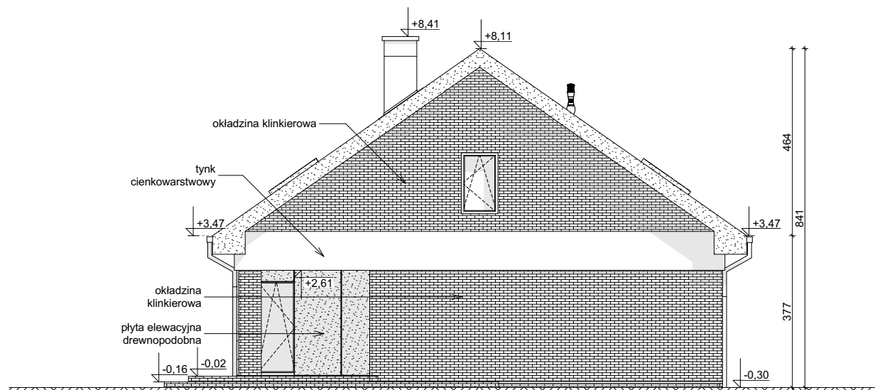
ELEWACJA BOCZNA
