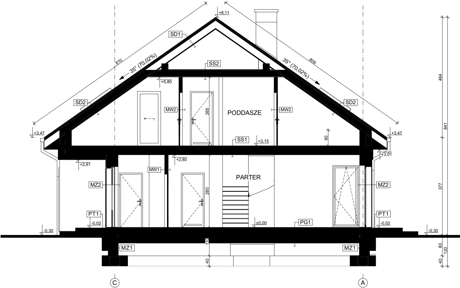
PRZEKRÓJ B-B
