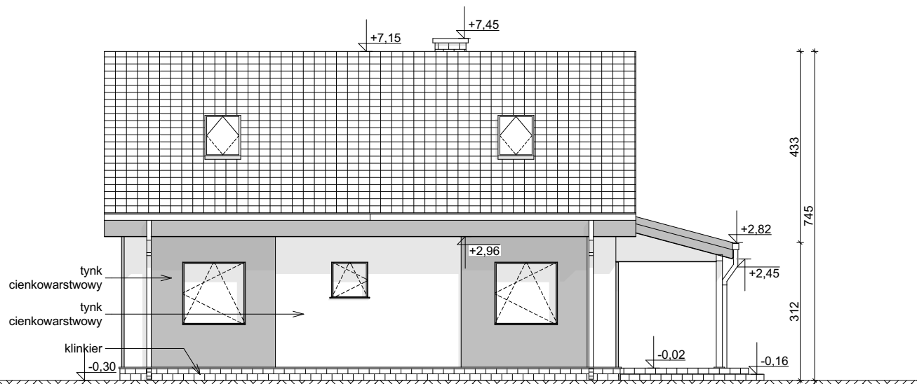
ELEWACJA OGRODOWA
