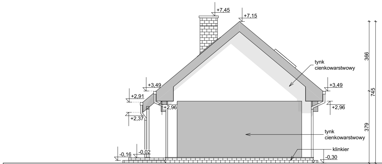
ELEWACJA BOCZNA
