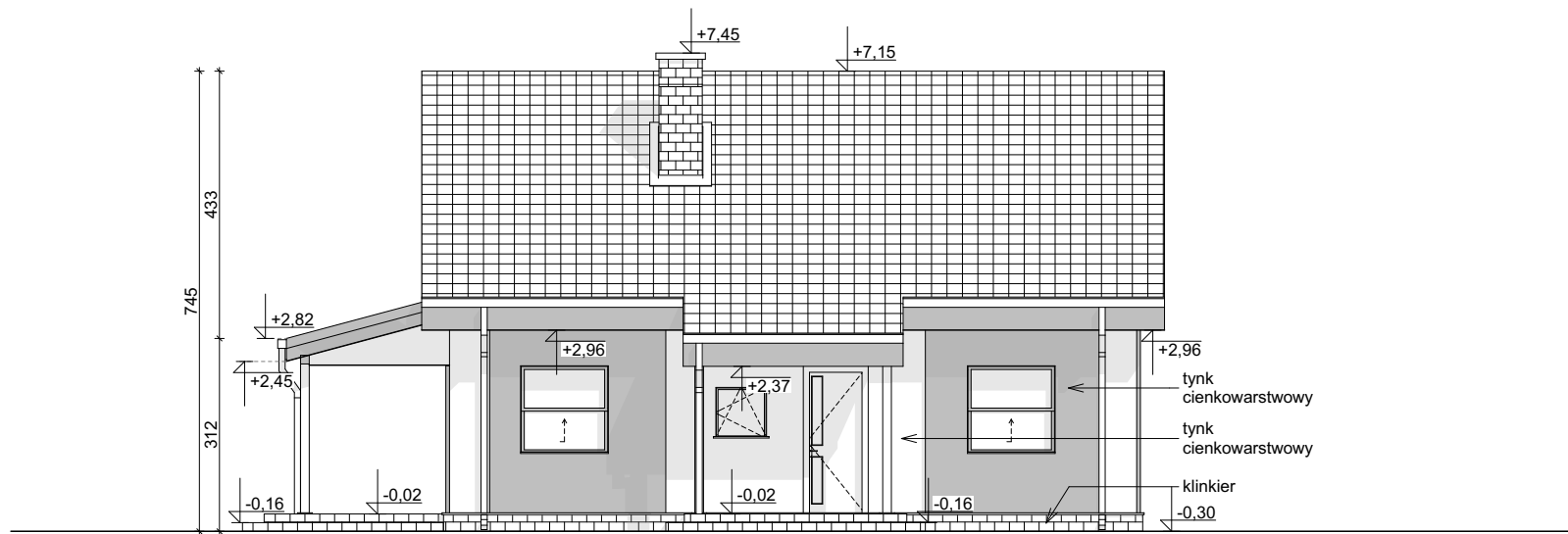
ELEWACJA FRONTOWA
