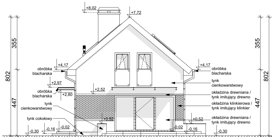
ELEVACJA BOCZNA
