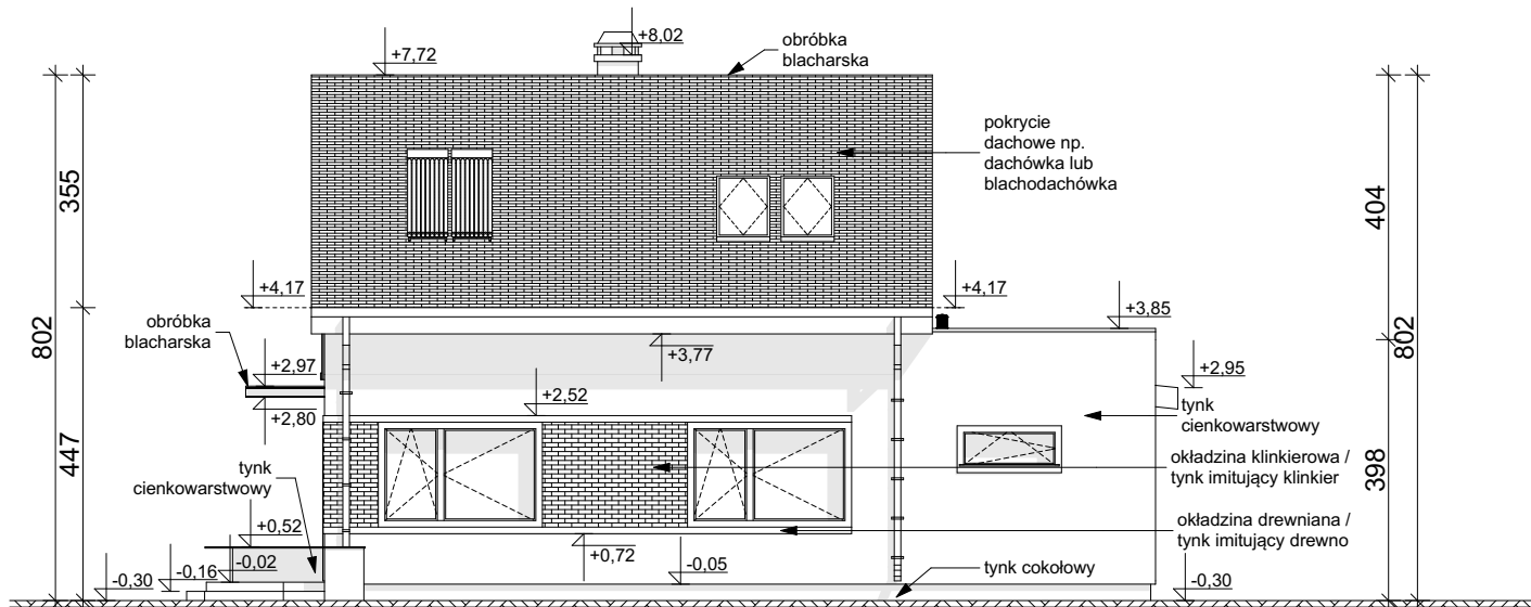
ELEVACJA OGRODOWA
