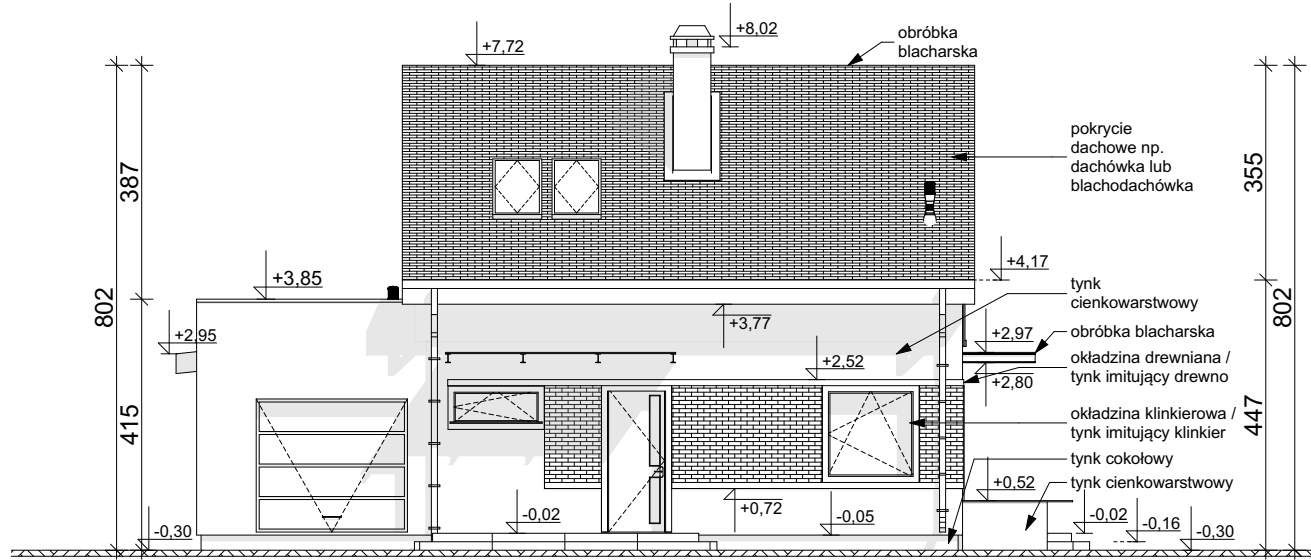
ELEWACJA FRONTOWA
