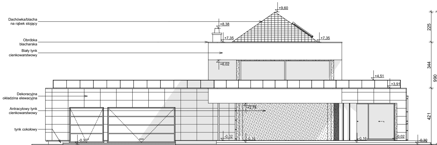
ELEWACJA BOCZNA
