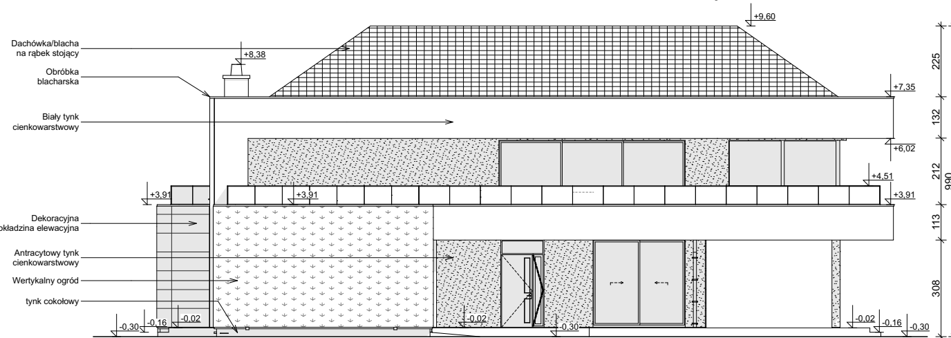
ELEWACJA FRONTOWA
