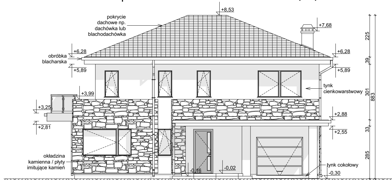
ELEWACJA FRONTOWA
