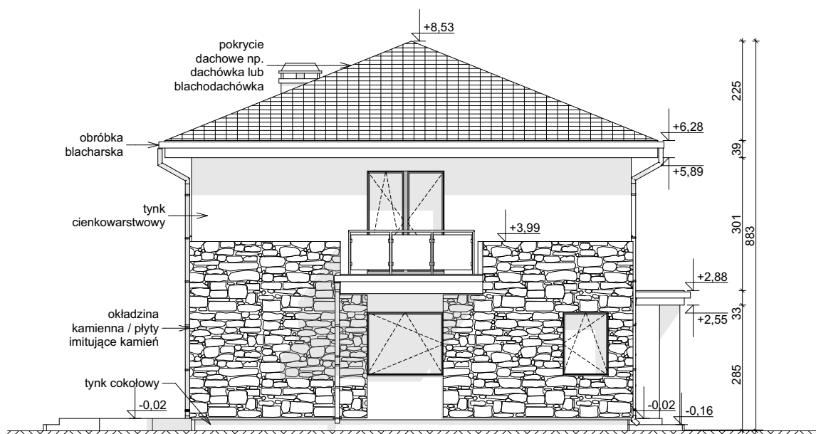
ELEWACJA BOCZNA
