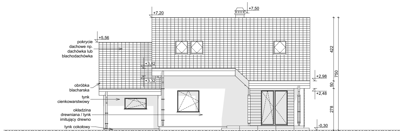
ELEWACJA OGRODOWA
