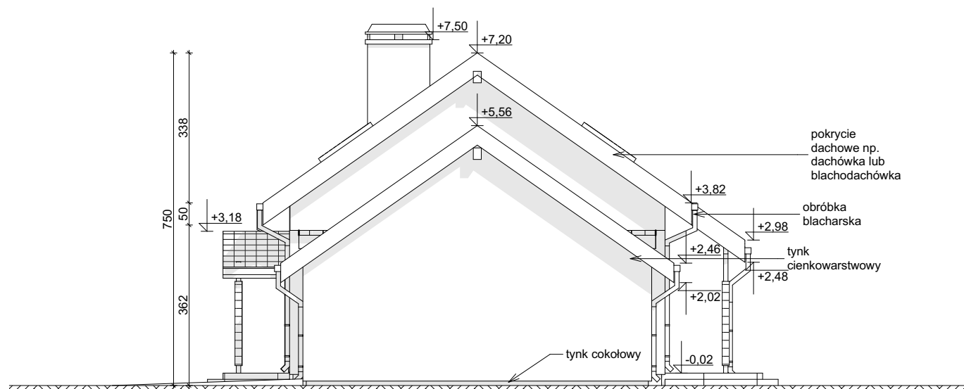
ELEWACJA BOCZNA
