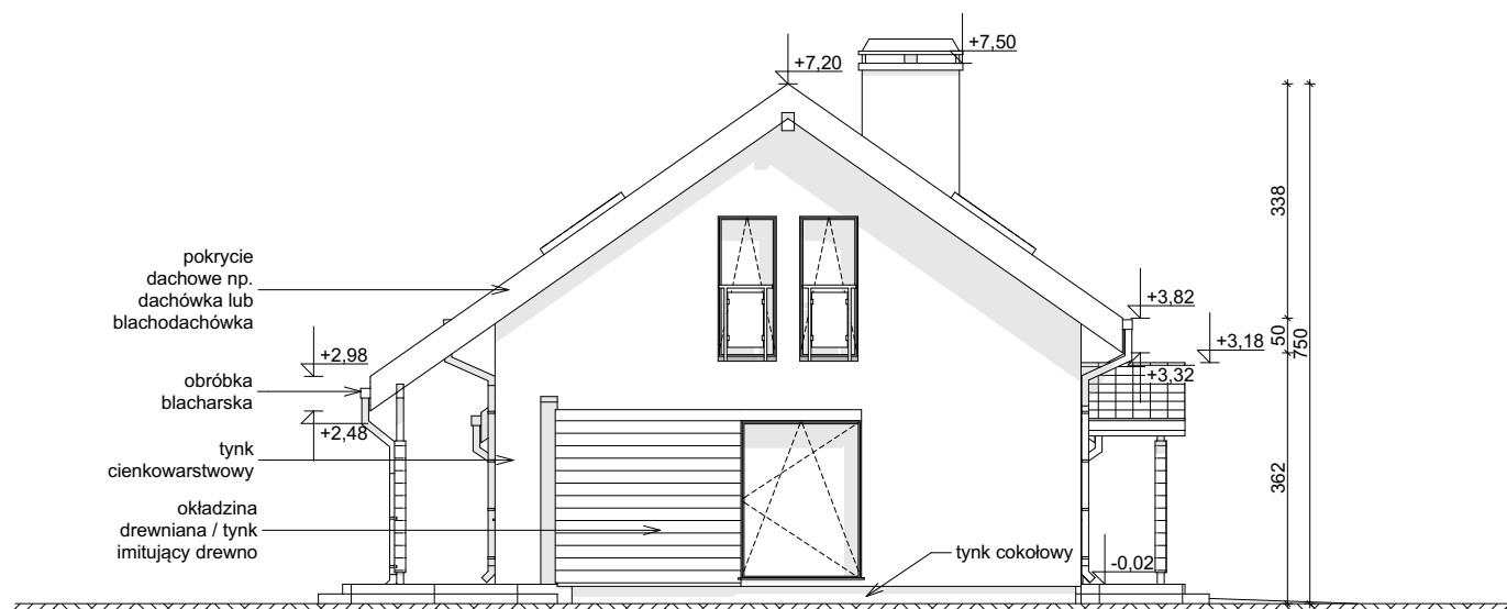
ELEWACJA BOCZNA
