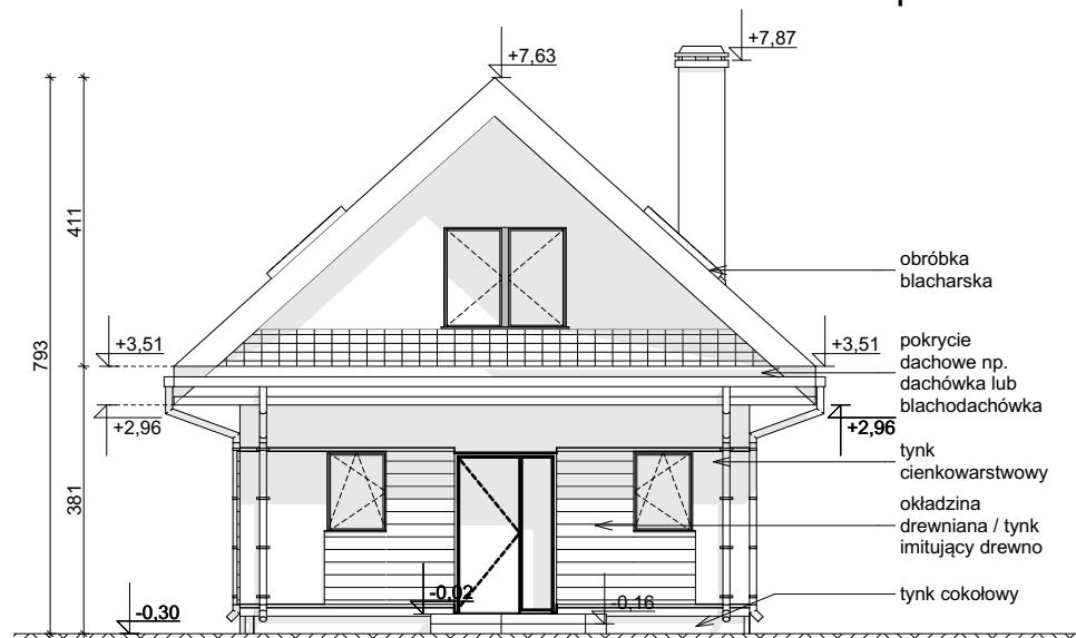
ELEWACJA FRONTOWA
