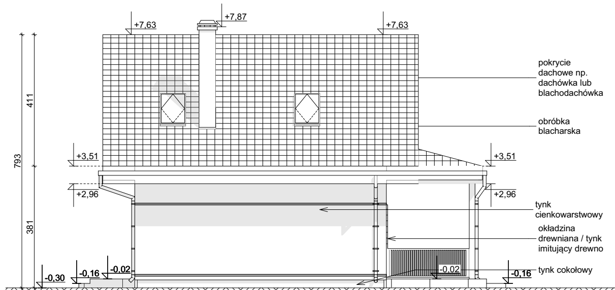
ELEWACJA BOCZNA
