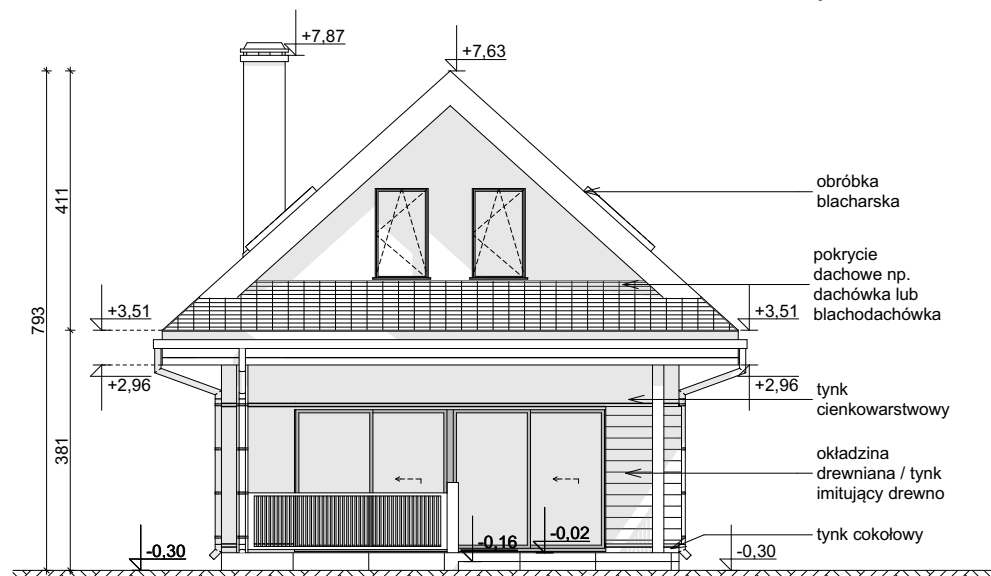
ELEWACJA OGRODOWA
