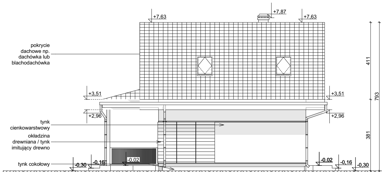
ELEWACJA BOCZNA
