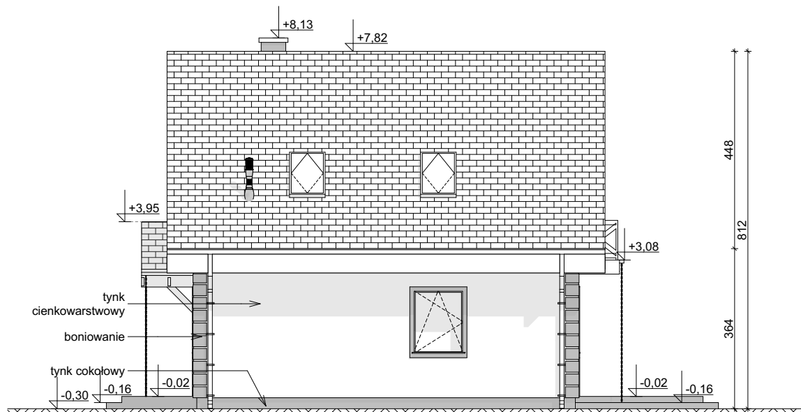
ELEWACJA BOCZNA
