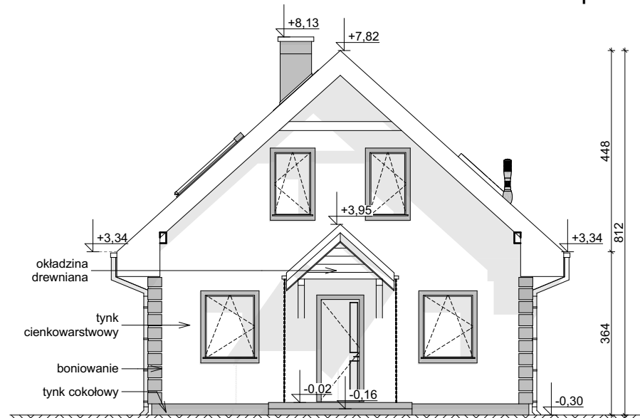
ELEWACJA FRONTOWA
