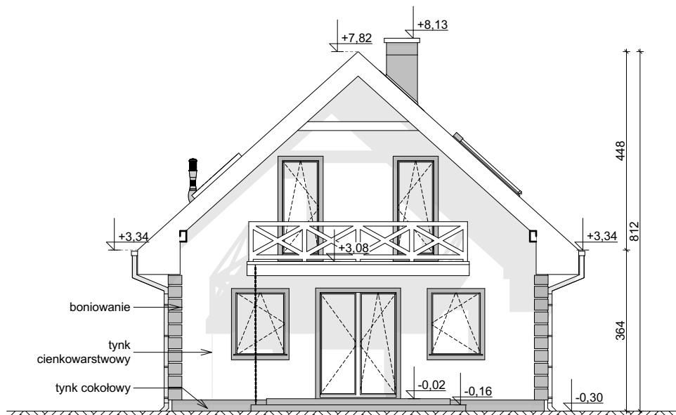
ELEWACJA OGRODOWA
