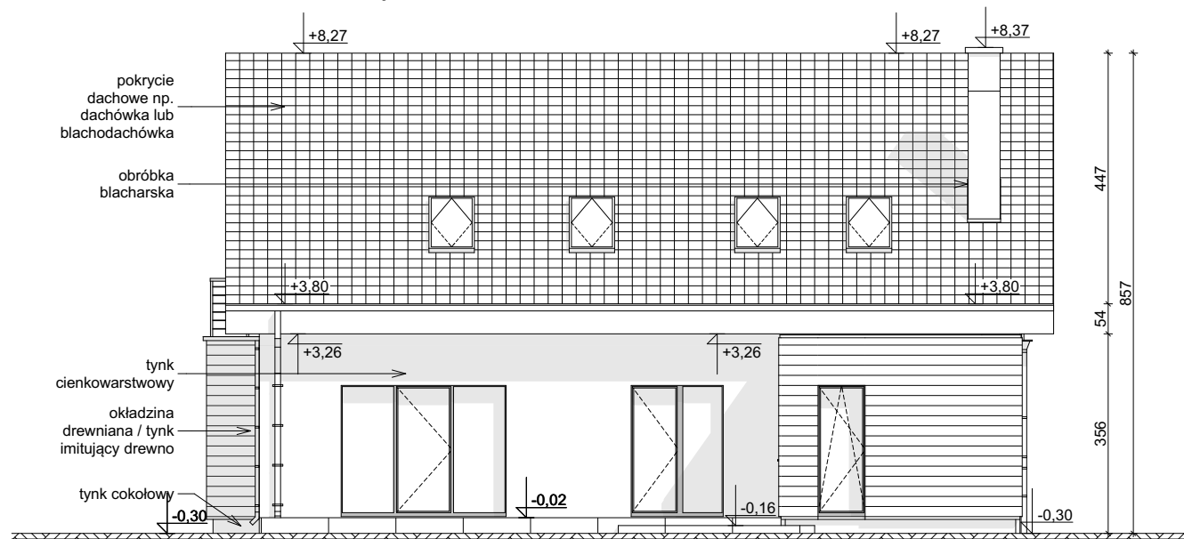
ELEWACJA OGRODOWA
