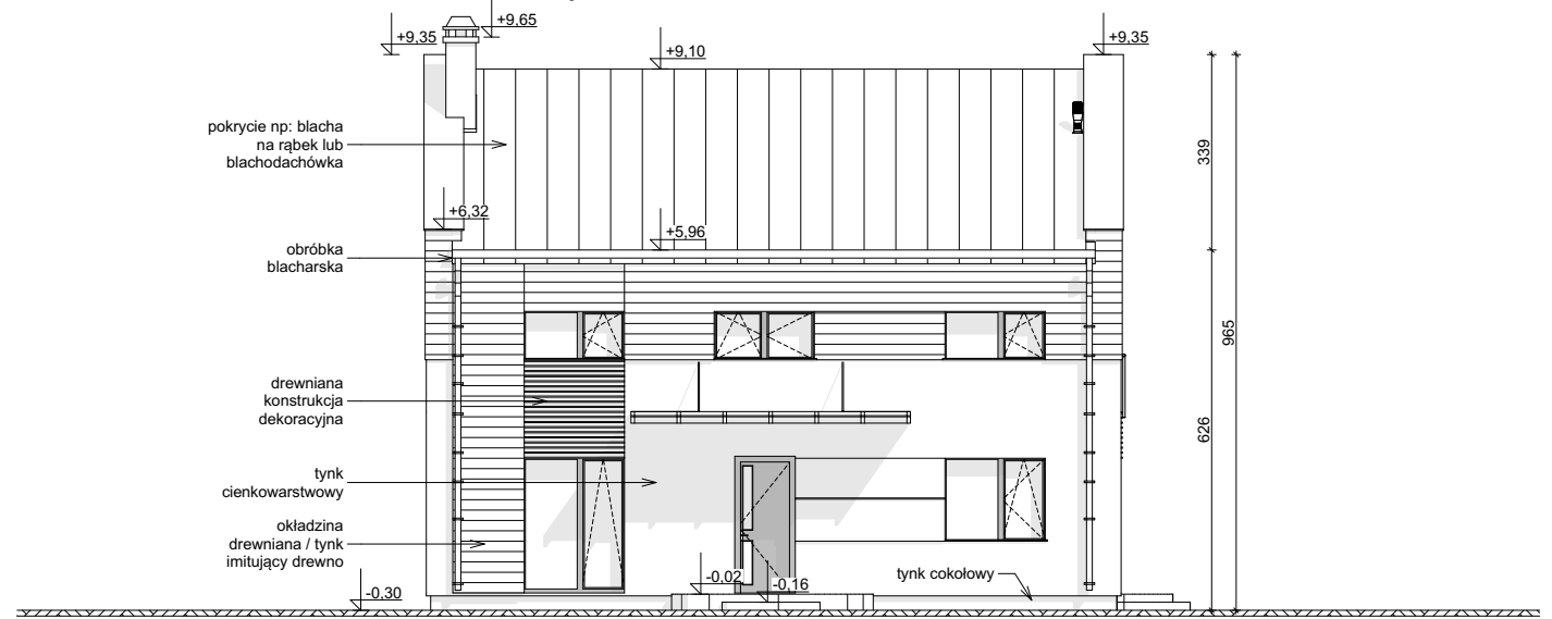
ELEWACJA FRONTOWA
