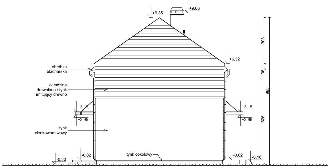
ELEWACJA BOCZNA
