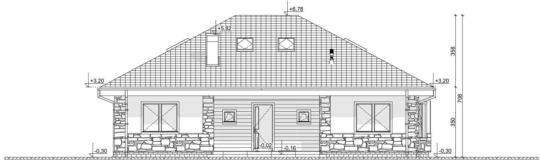
ELEWACJA FRONTOWA
