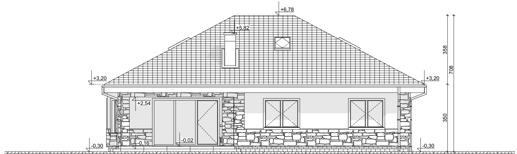
ELEWACJA OGRODOWA
