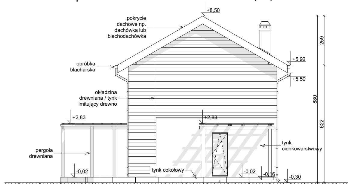
ELEWACJA OGRODOWA
