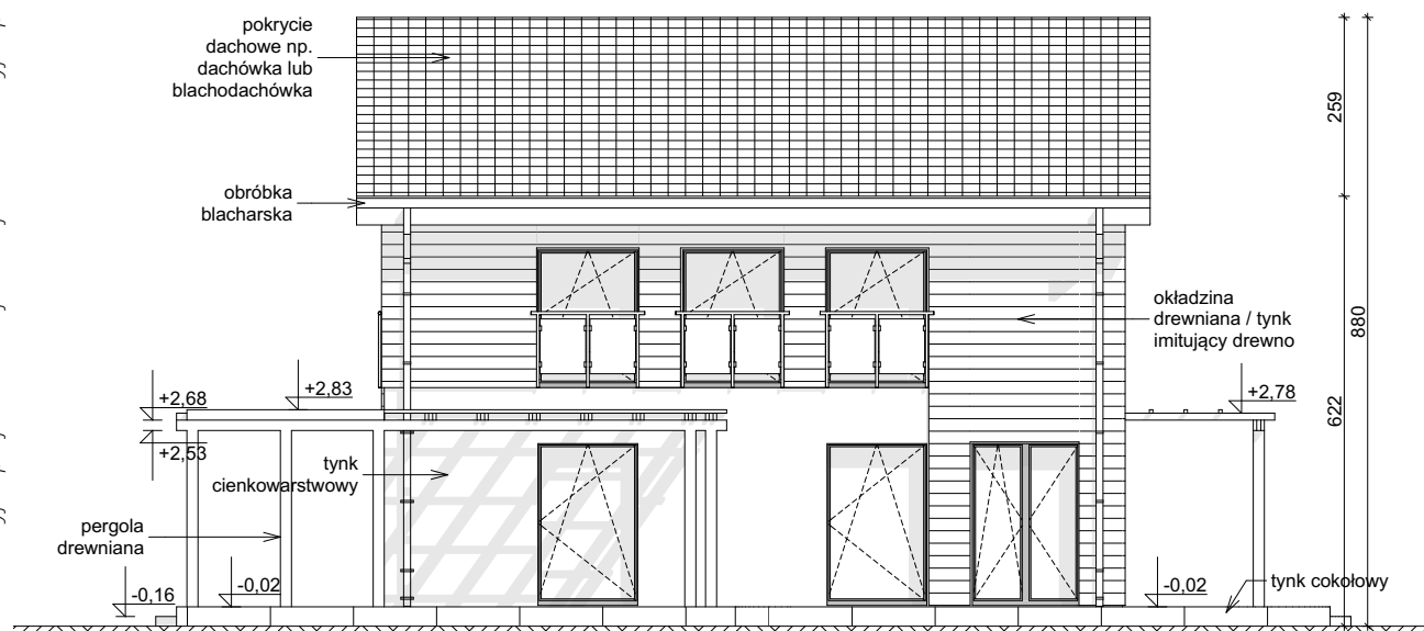
ELEWACJA BOCZNA
