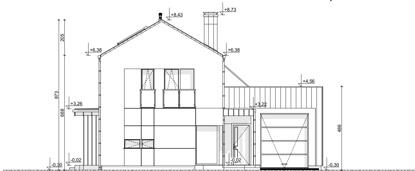
ELEWACJA FRONTOWA
