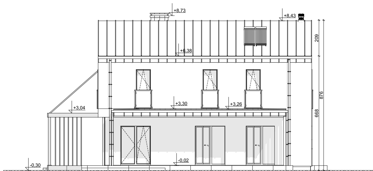
ELEWACJA BOCZNA
