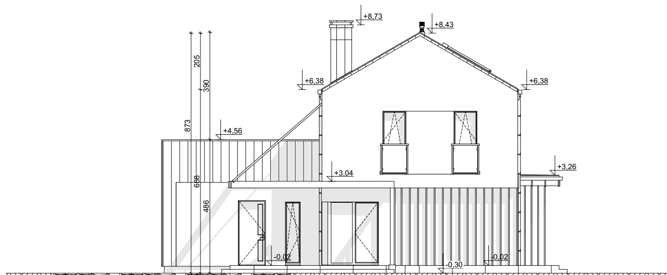
ELEWACJA OGRODOWA
