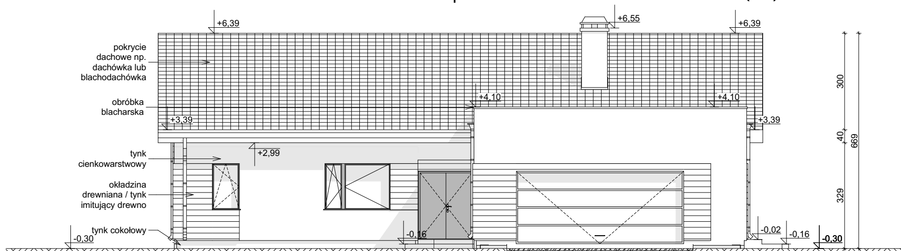
ELEWACJA FRONTOWA
