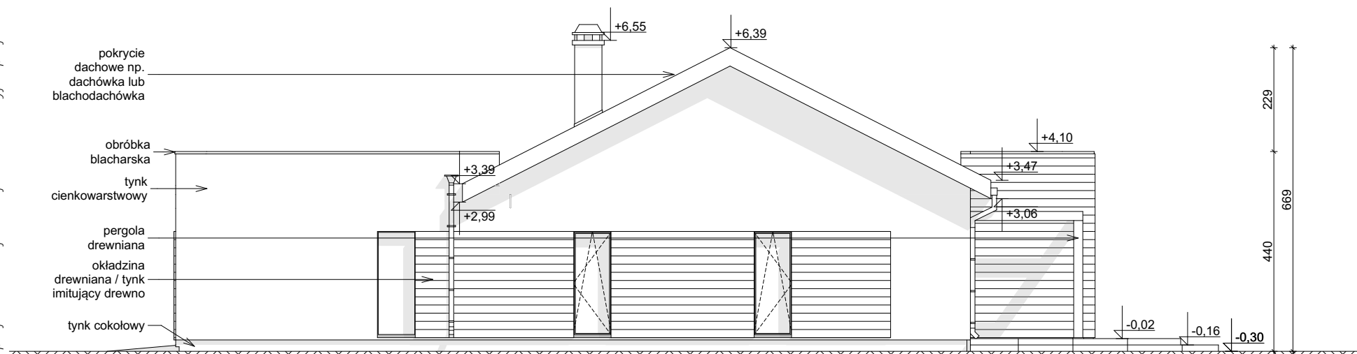
ELEWACJA BOCZNA
