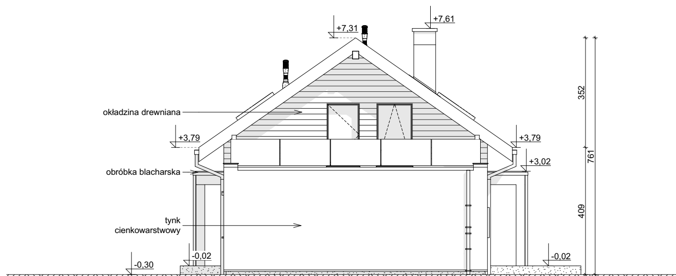
ELEWACJA BOCZNA
