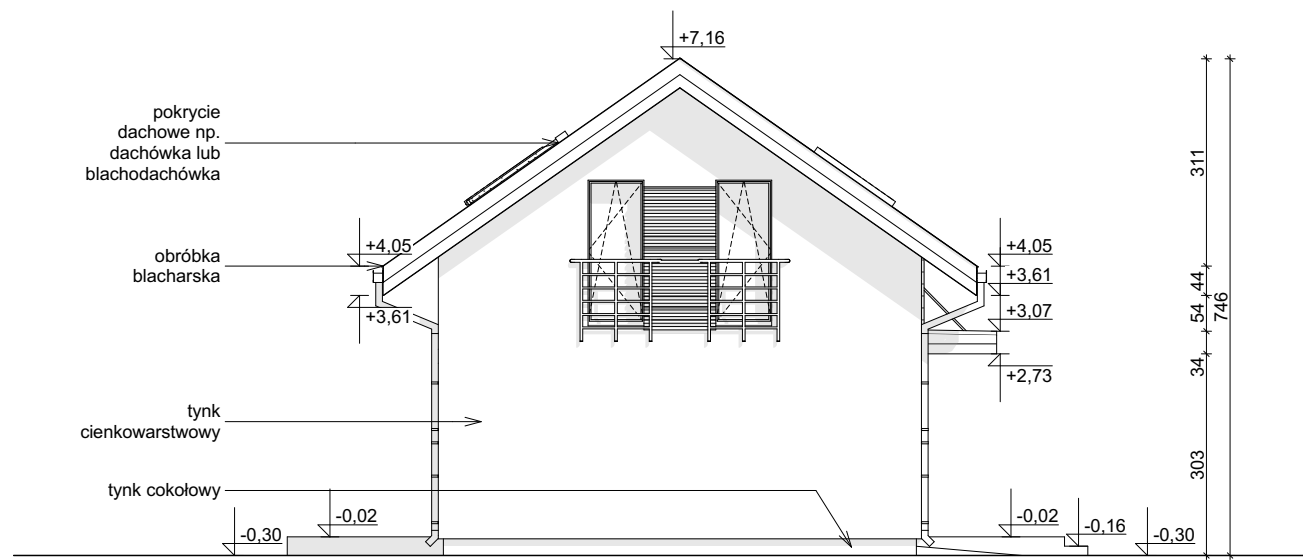
ELEWACJA BOCZNA
