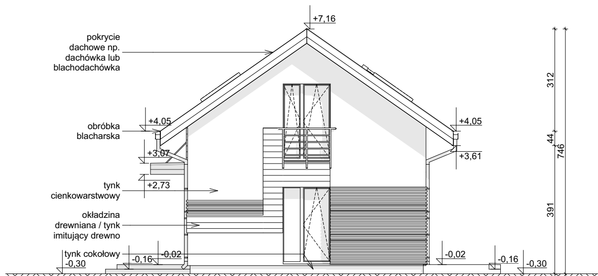
ELEWACJA BOCZNA
