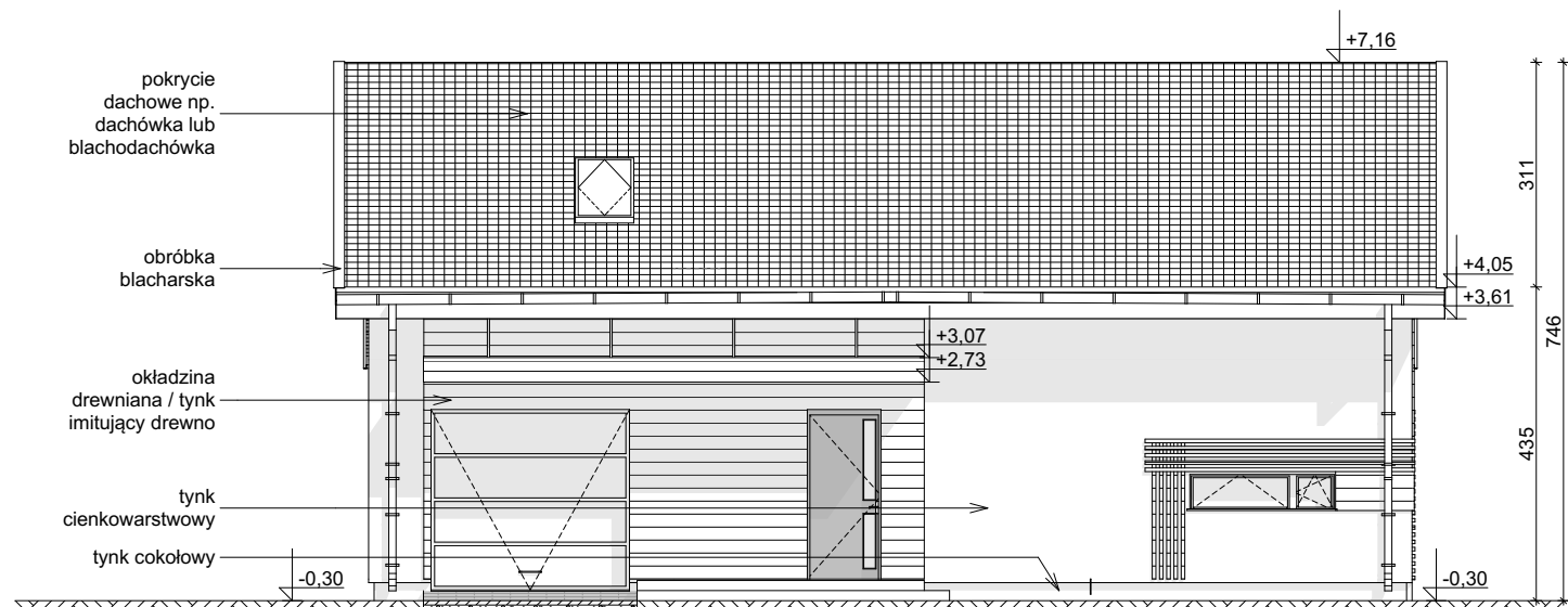
ELEWACJA FRONTOWA
