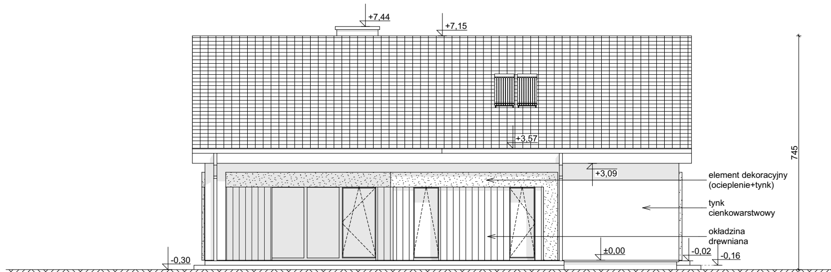
ELEWACJA BOCZNA
