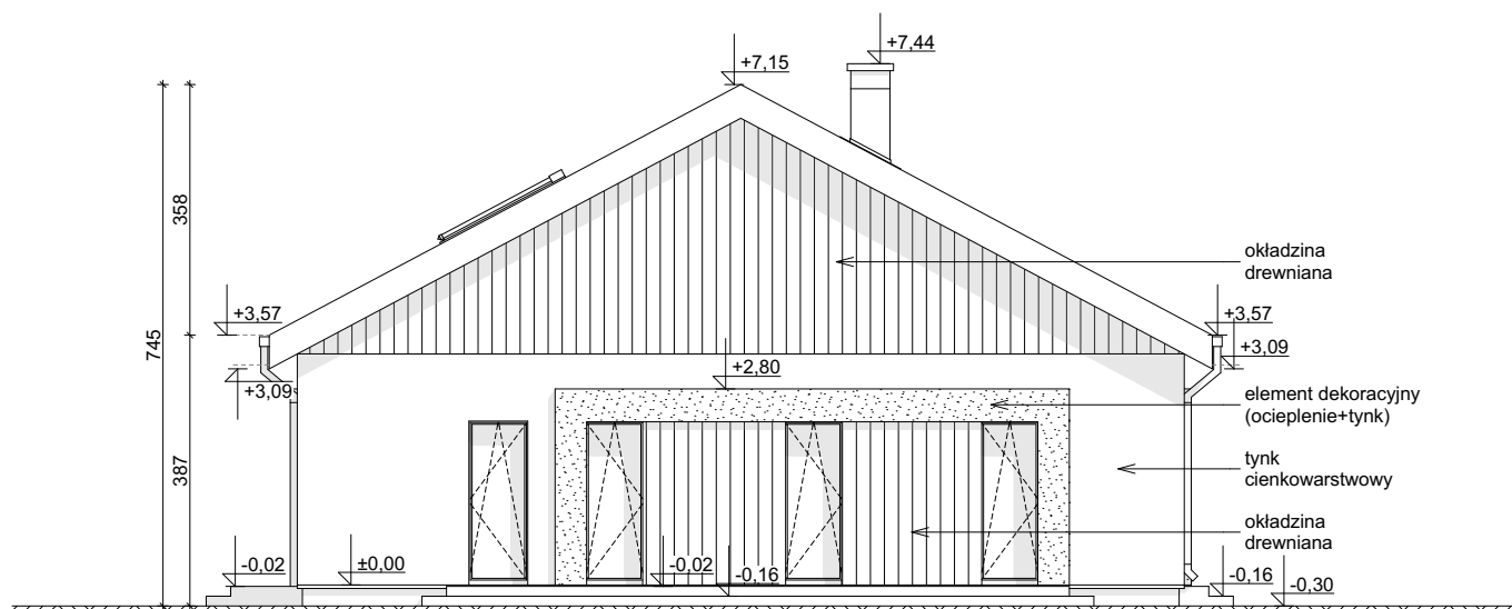
ELEWACJA BOCZNA
