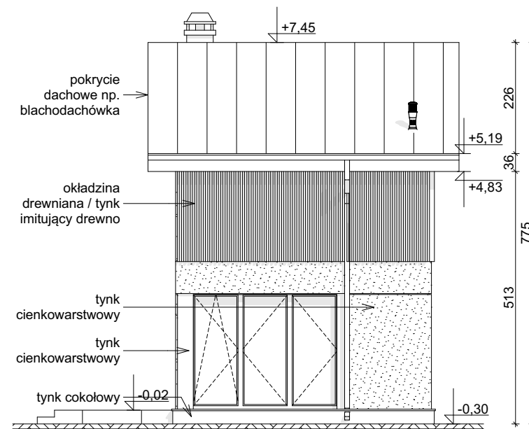
ELEWACJA OGRODOWA
