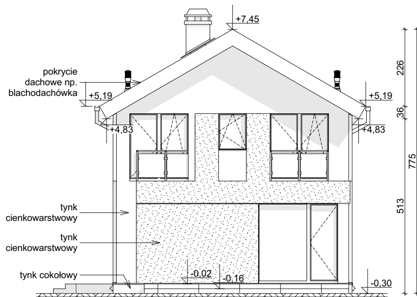
ELEWACJA BOCZNA
