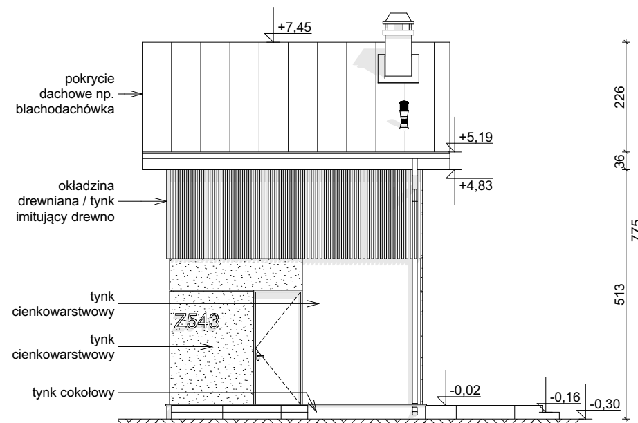
ELEWACJA FRONTOWA
