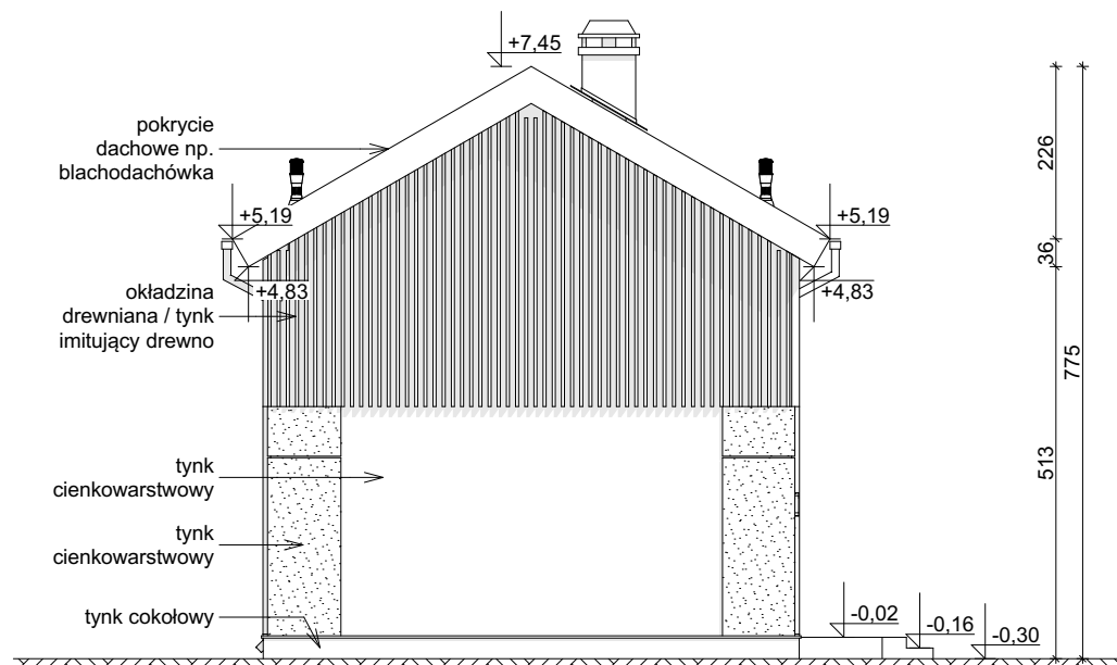
ELEWACJA BOCZNA
