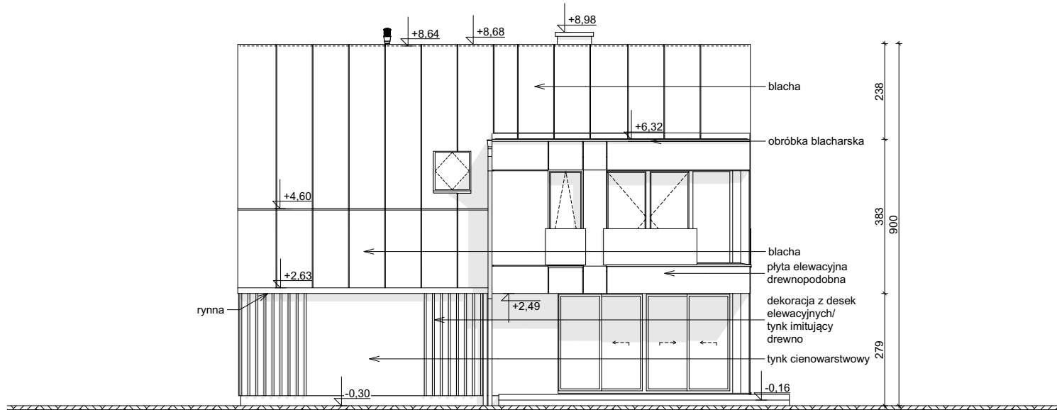
ELEWACJA OGRODOWA
