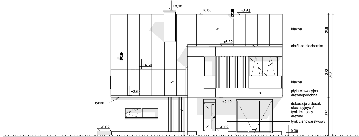
ELEWACJA FRONTOWA
