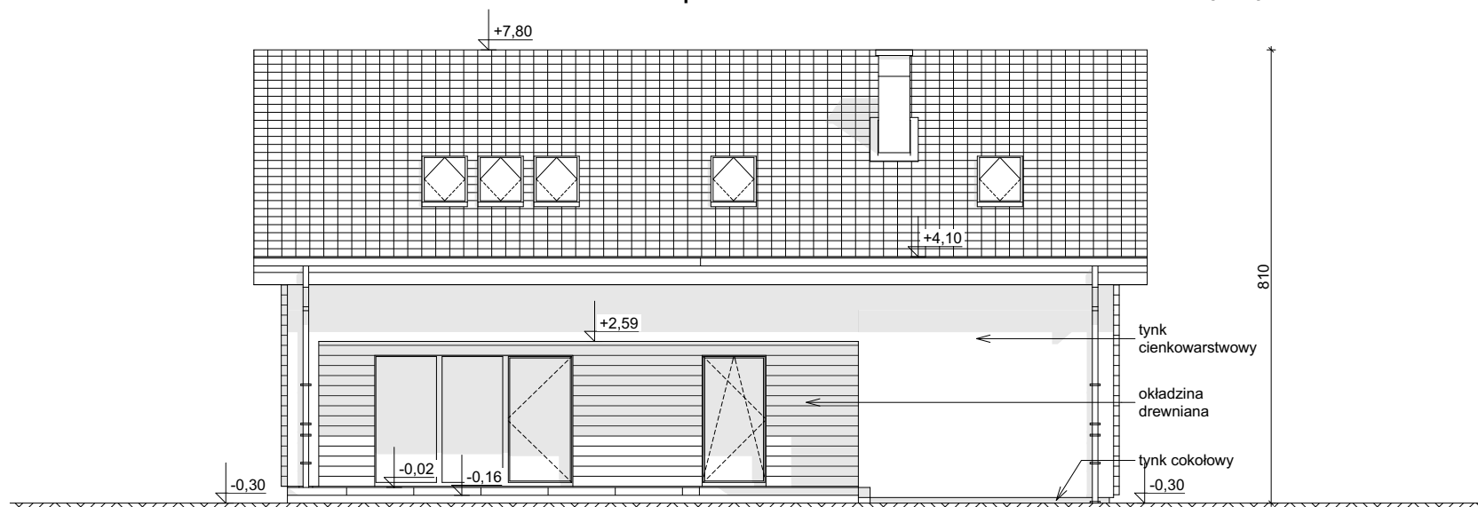
ELEWACJA OGRODOWA
