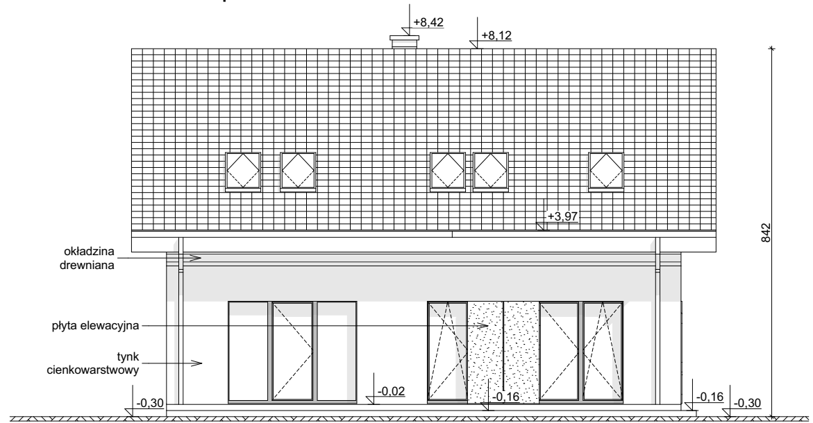
ELEWACJA OGRODOWA
