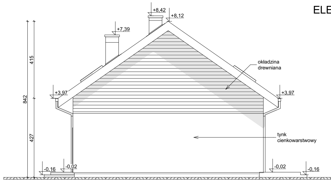
ELEWACJA BOCZNA
