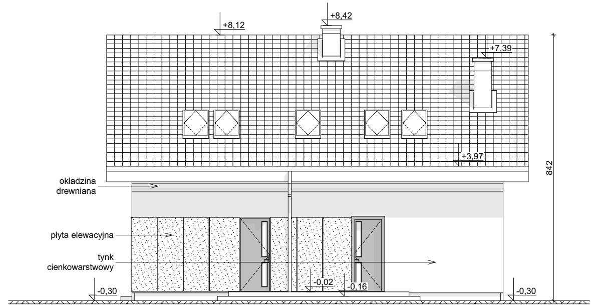
ELEWACJA FRONTOWA
