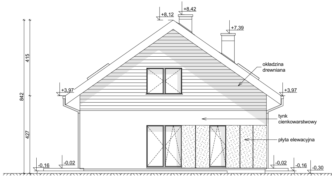
ELEWACJA BOCZNA
