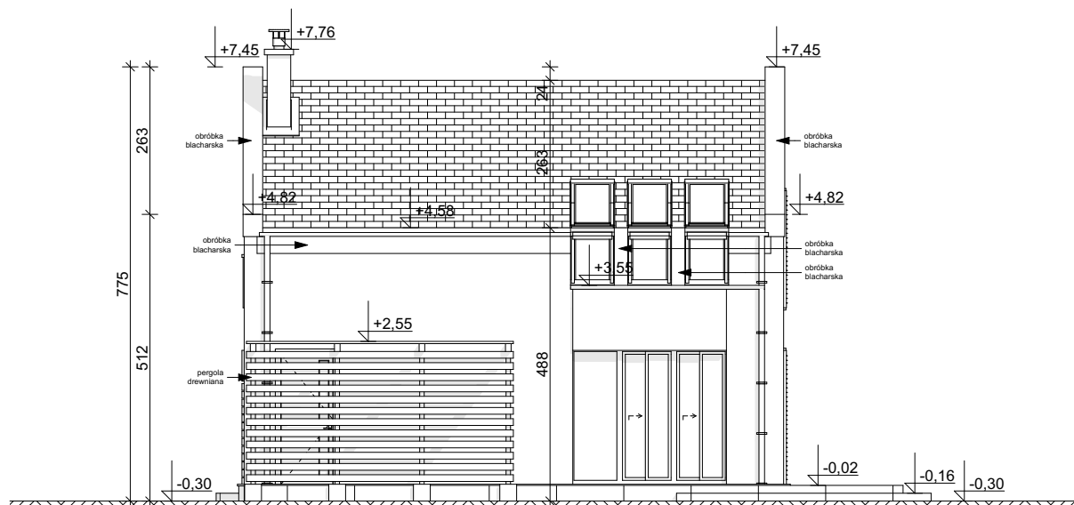
ELEWACJA OGRODOWA
