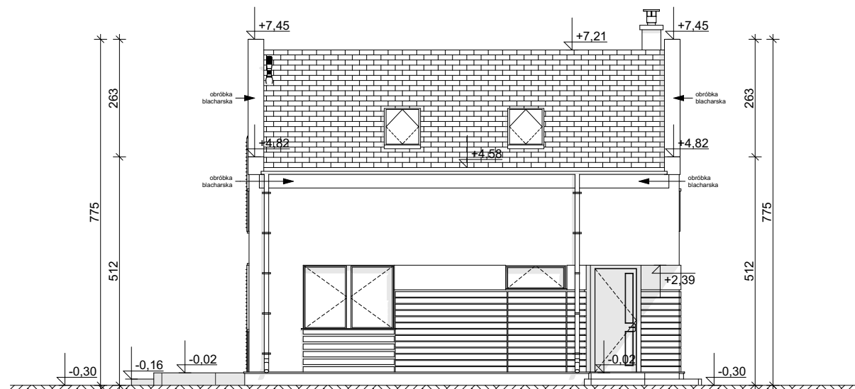
ELEWACJA FRONTOWA
