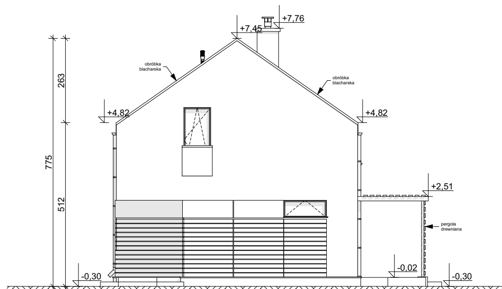
ELEWACJA BOCZNA
