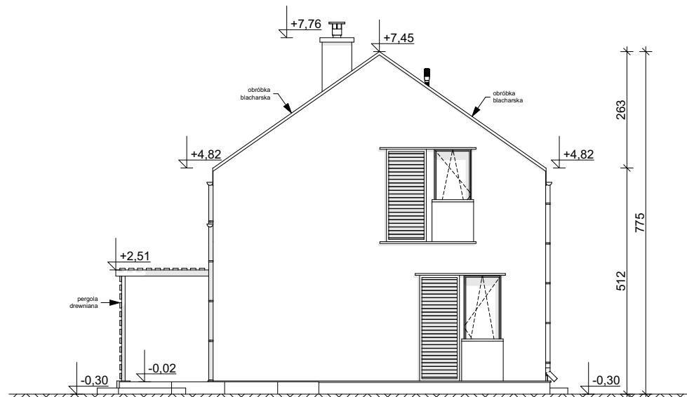
ELEWACJA BOCZNA
