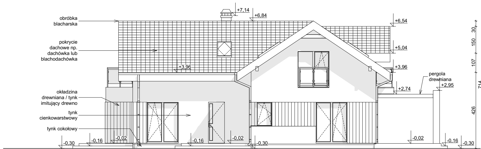
ELEWACJA FRONTOWA
