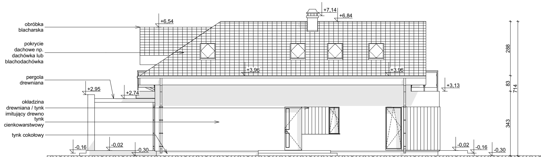
ELEWACJA OGRODOWA
