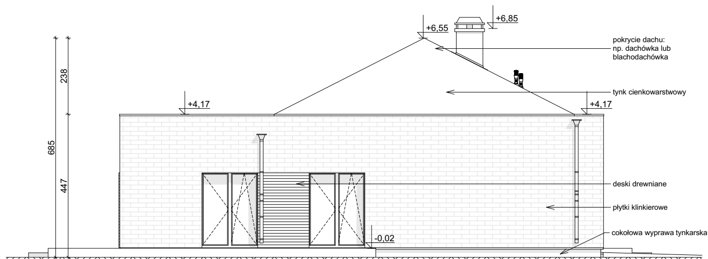
ELEWACJA BOCZNA
