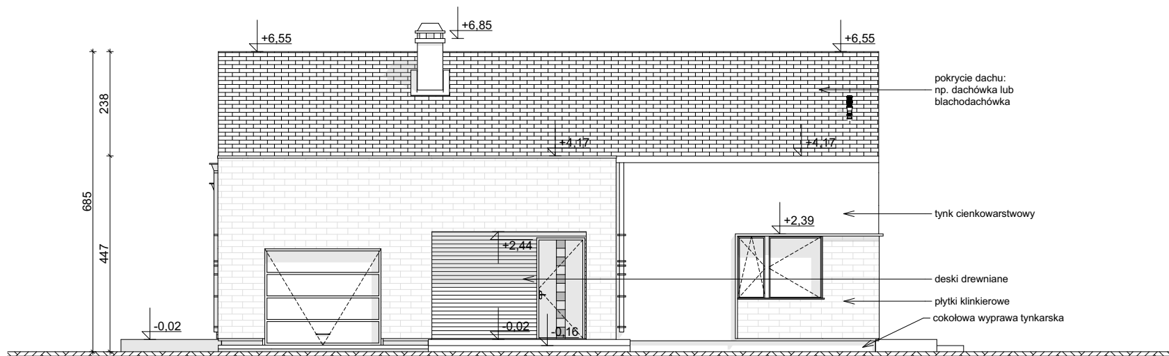
ELEWACJA FRONTOWA
