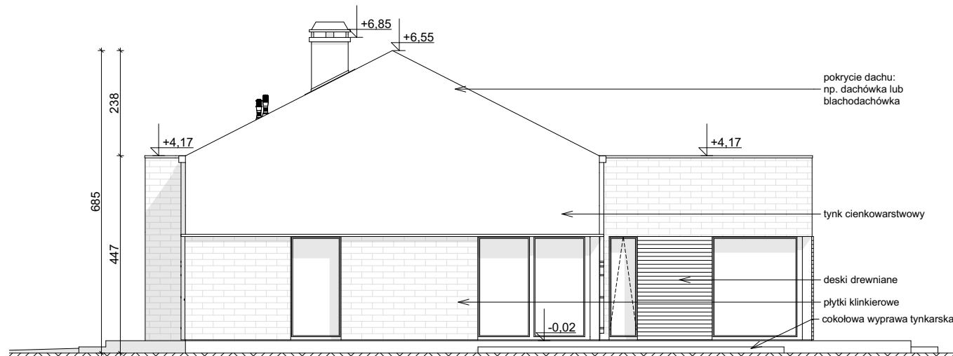
ELEWACJA BOCZNA
