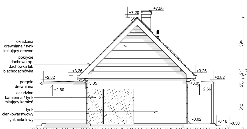
ELEWACJA BOCZNA
