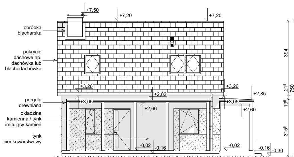
ELEWACJA FRONTOWA
