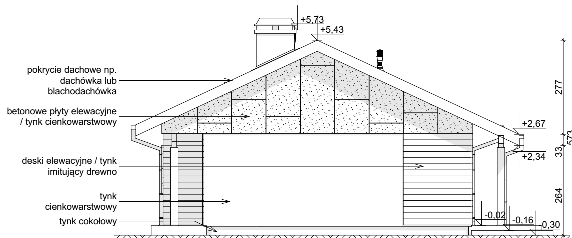
ELEWACJA BOCZNA
