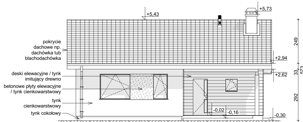
ELEWACJA FRONTOWA
