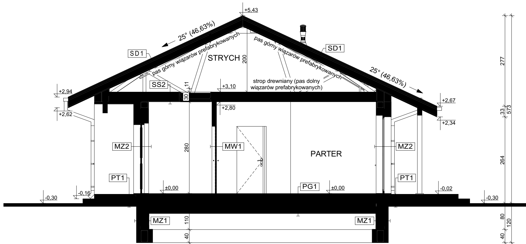
PRZEKRÓJ B-B
