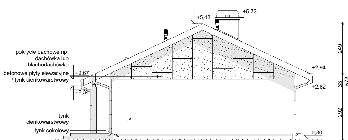
ELEWACJA BOCZNA
