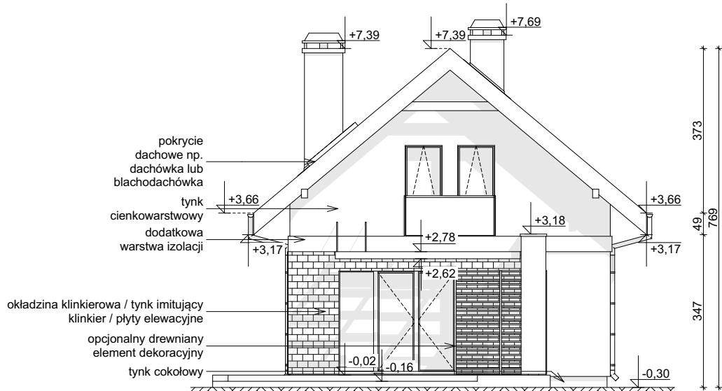
ELEWACJA OGRODOWA
