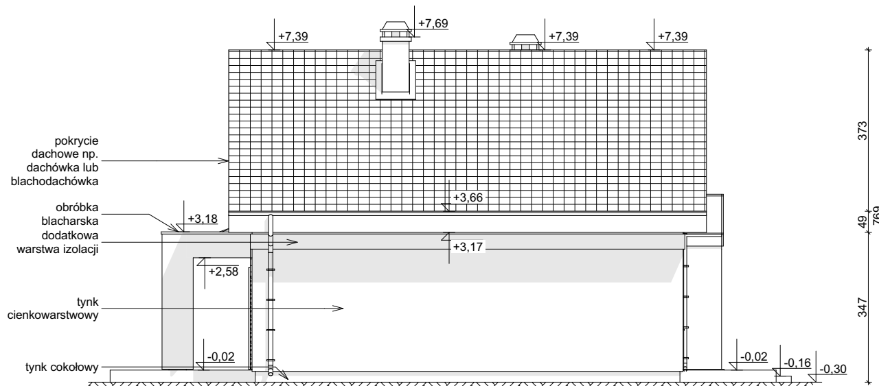
ELEWACJA BOCZNA
