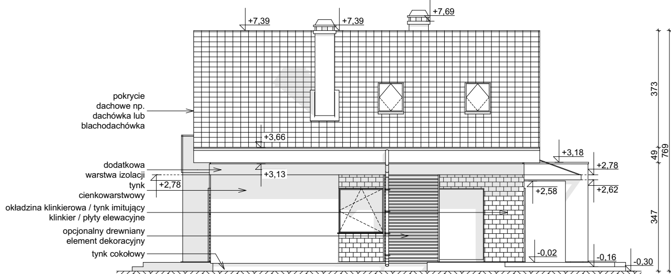
ELEWACJA BOCZNA
