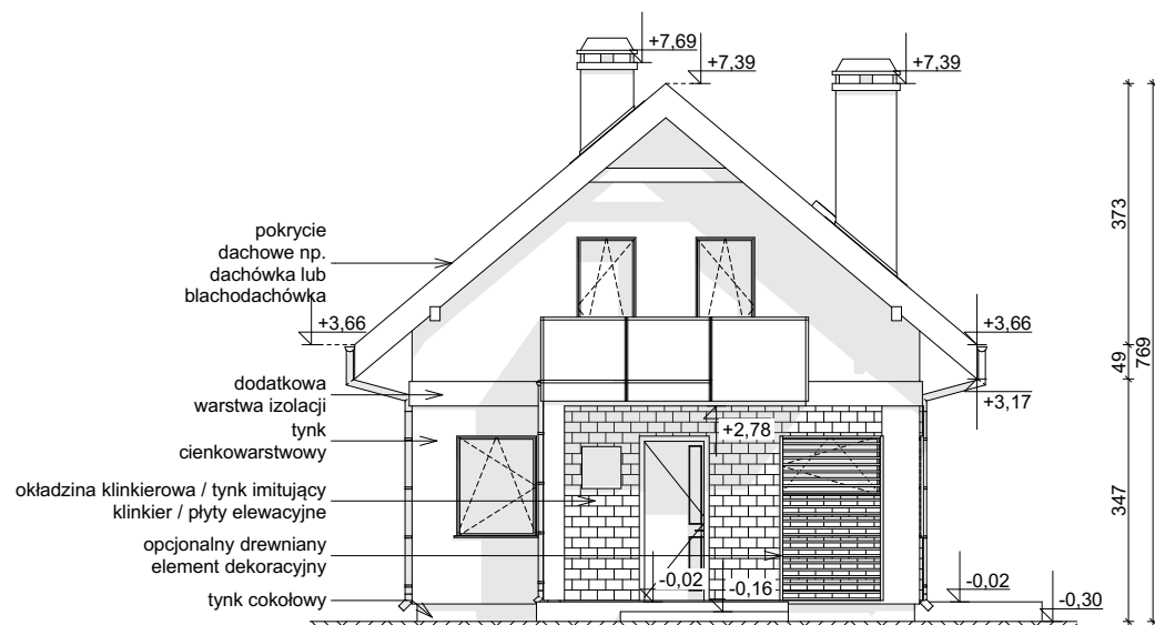
ELEWACJA FRONTOWA
