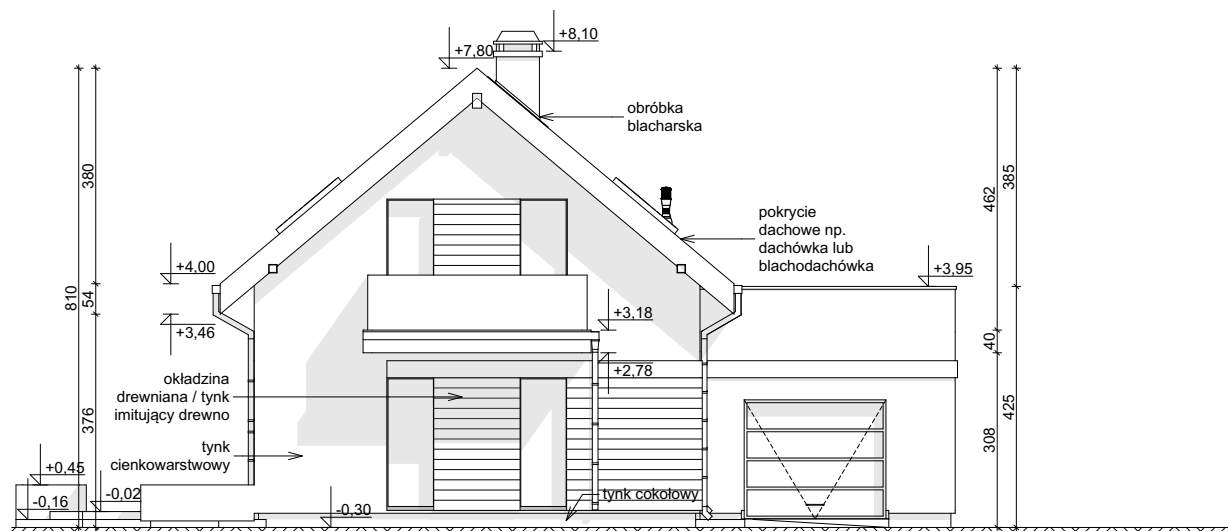
ELEWACJA BOCZNA
