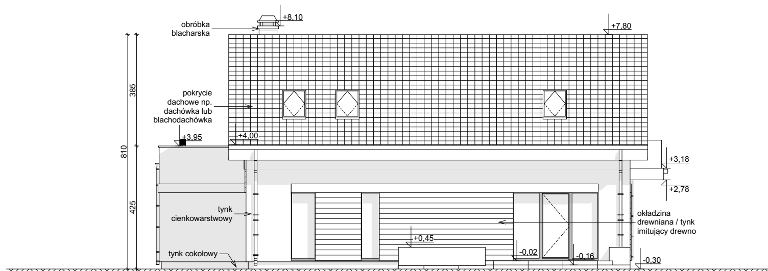
ELEWACJA OGRODOWA
