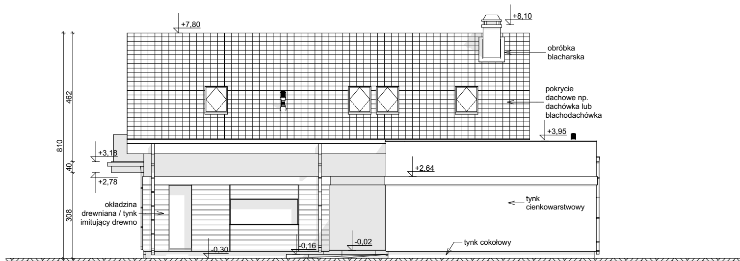
ELEWACJA FRONTOWA
