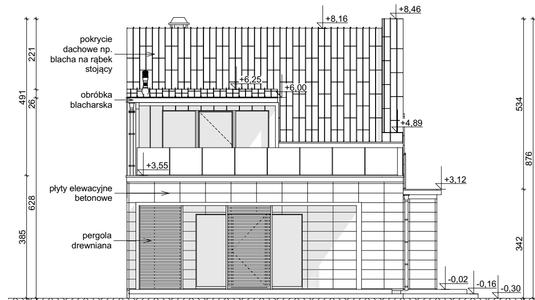
ELEWACJA OGRODOWA
