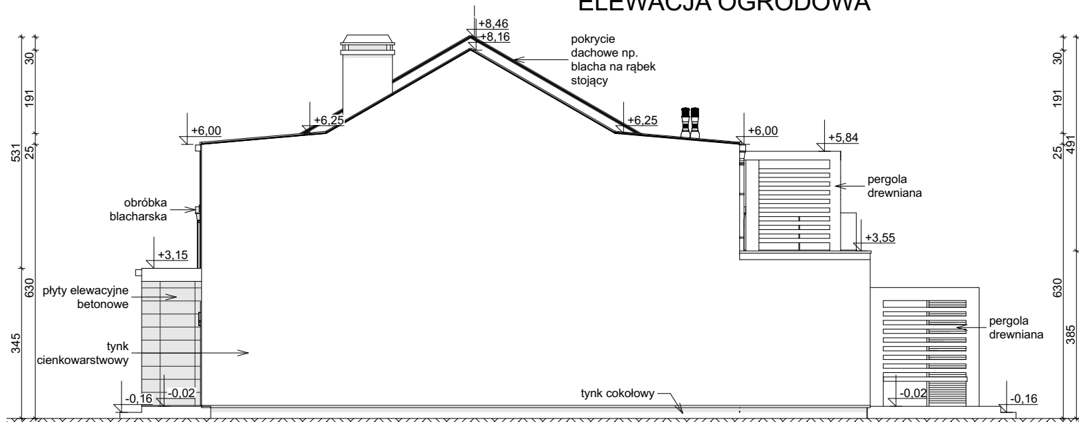
ELEWACJA BOCZNA
