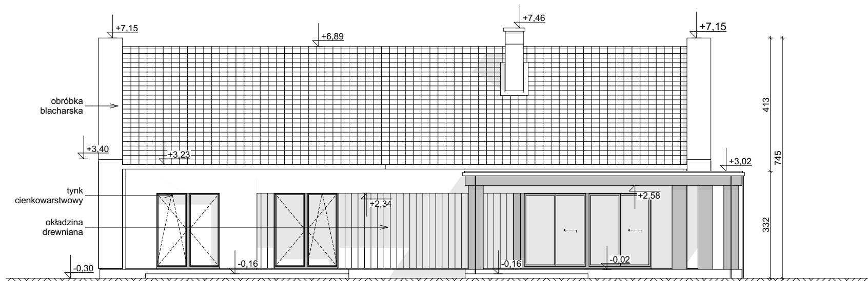
ELEWACJA OGRODOWA
