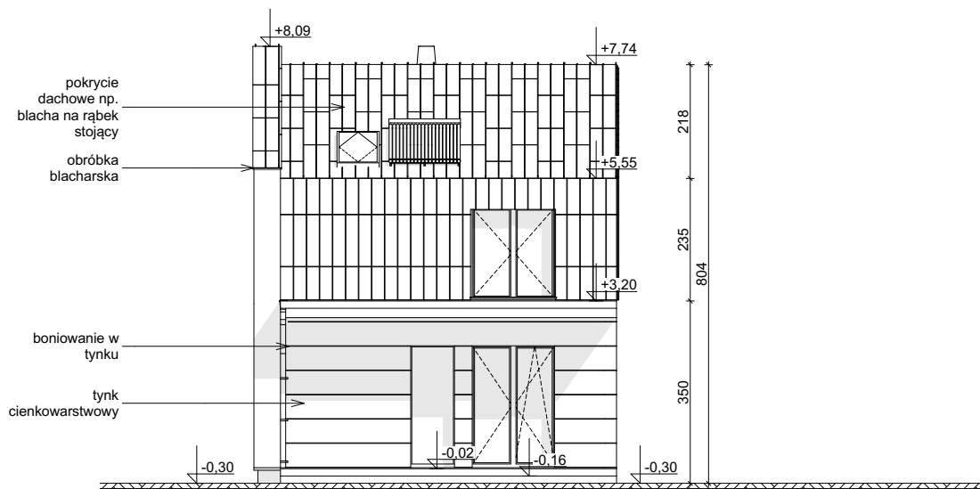
ELEVACJA OGRODOWA
