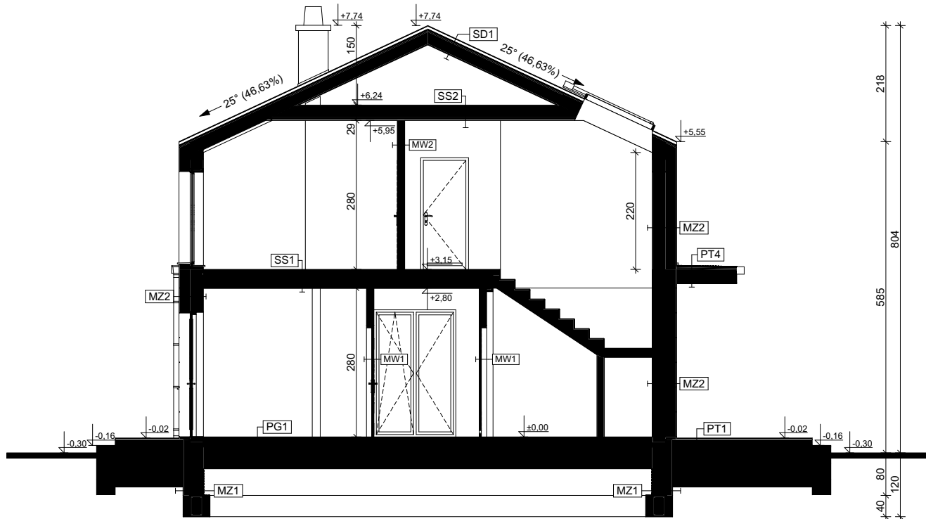
B-B PRZEKRÓJ
