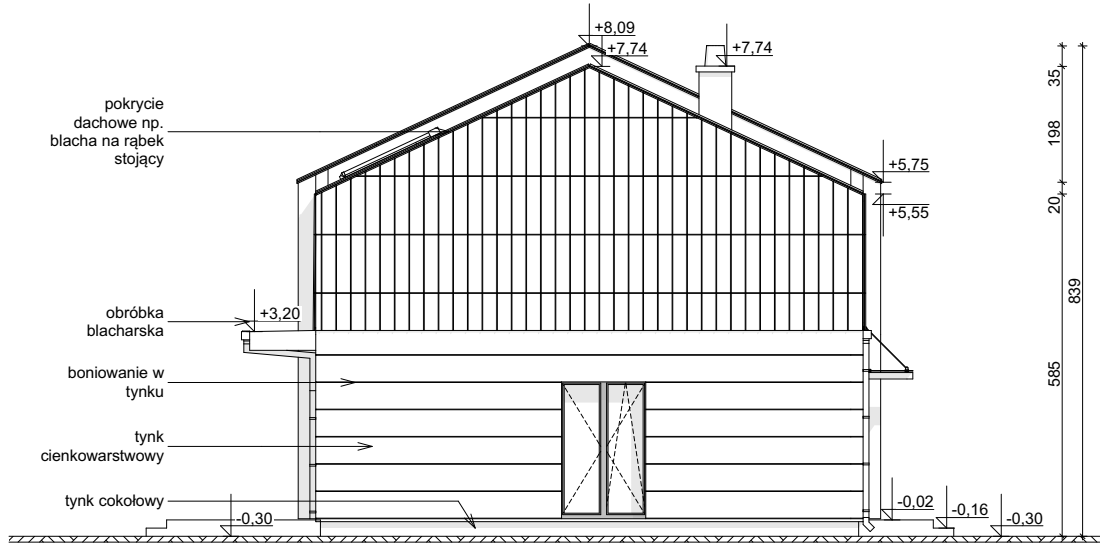
ELEVACJA BOCZNA
