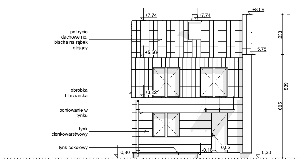
ELEWACJA FRONTOWA
