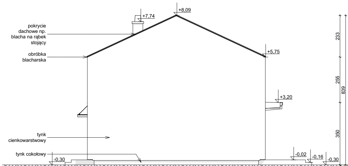
ELEWACJA BOCZNA
