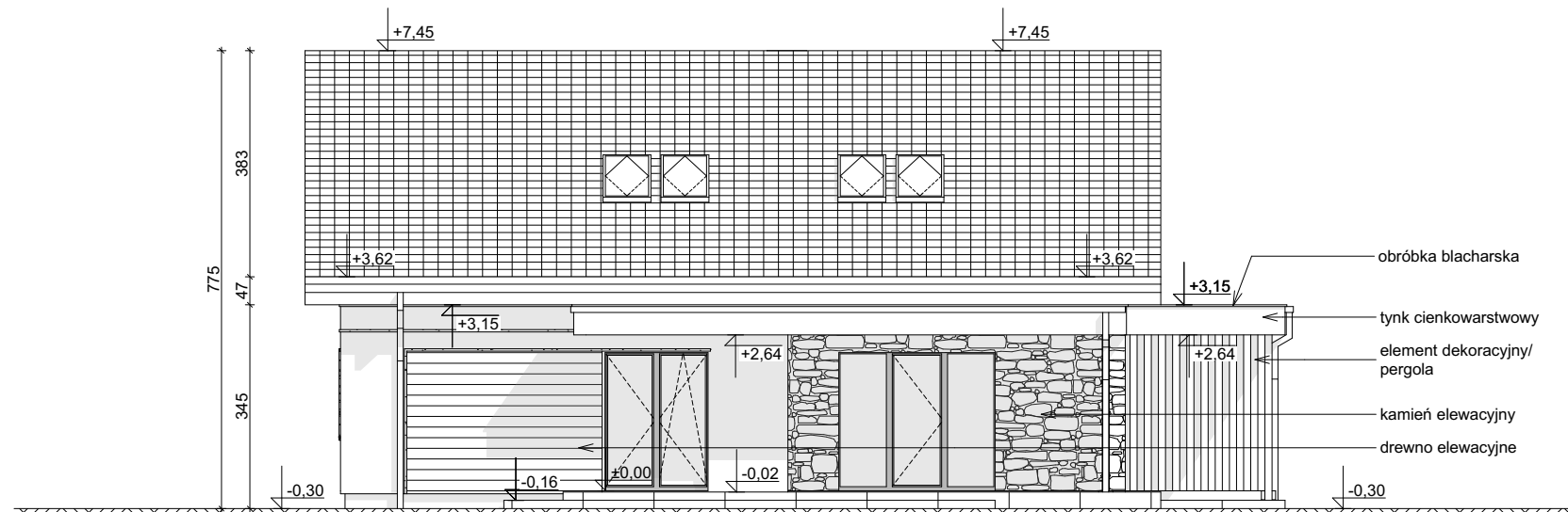
ELEWACJA OGRODOWA
