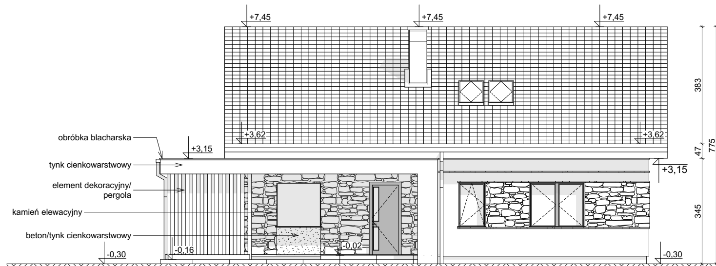
ELEWACJA FRONTOWA
