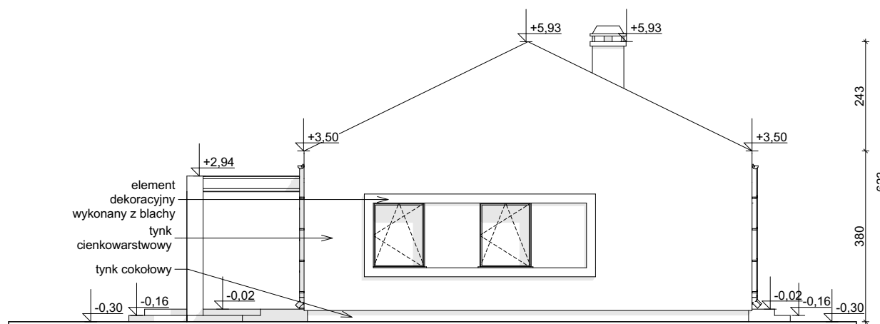
ELEWACJA BOCZNA
