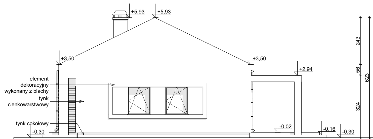
ELEWACJA BOCZNA
