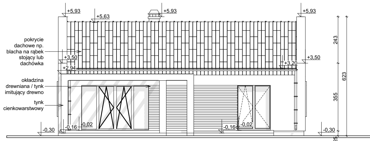
ELEWACJA OGRODOWA
