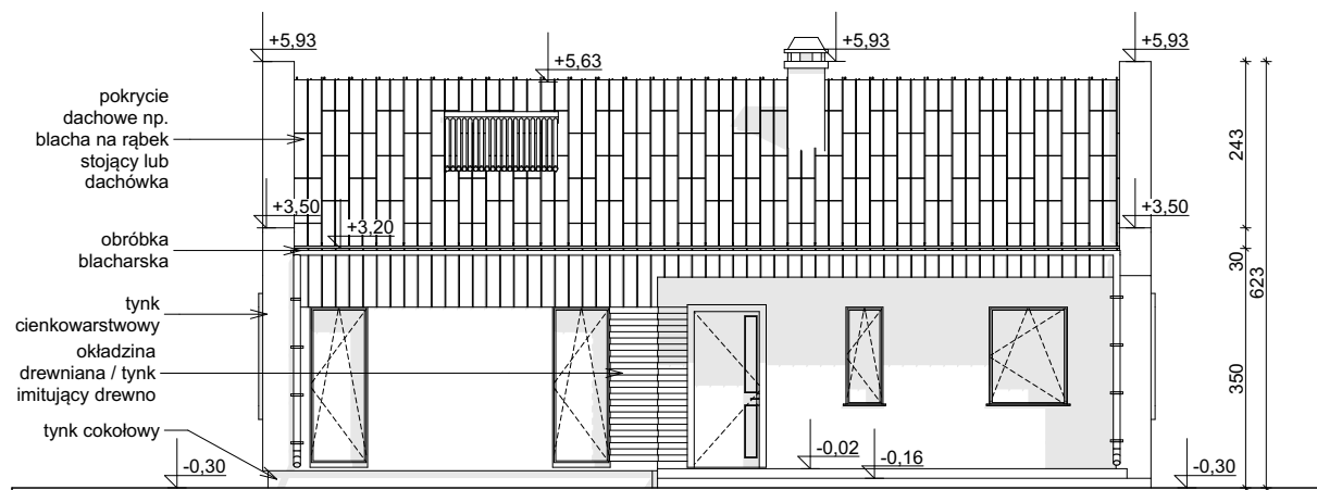
ELEWACJA FRONTOWA
