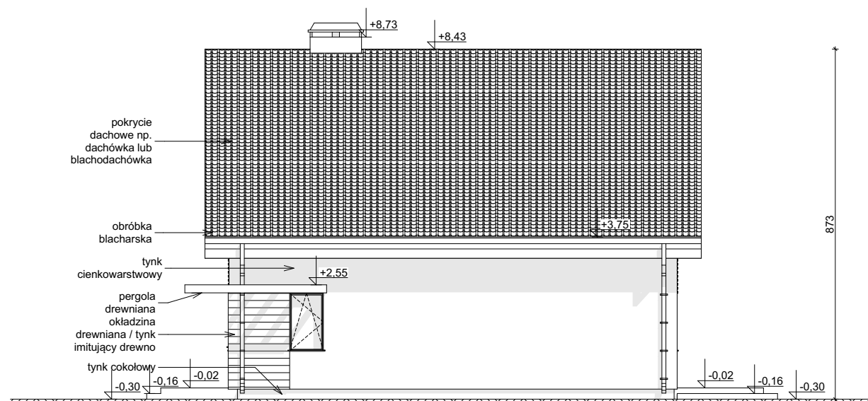
ELEWACJA BOCZNA
