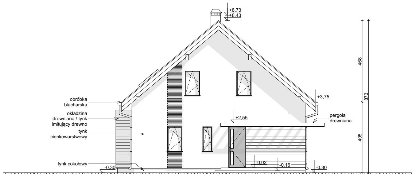
ELEWACJA FRONTOWA
