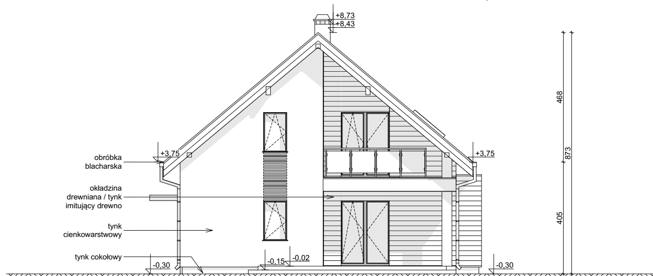
ELEWACJA OGRODOWA
