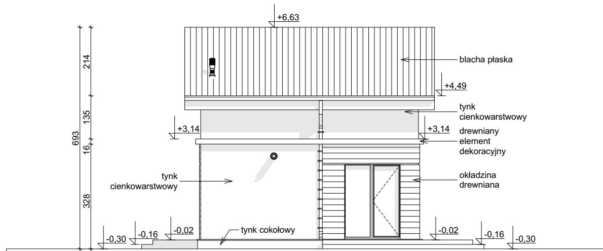
ELEWACJA BOCZNA
