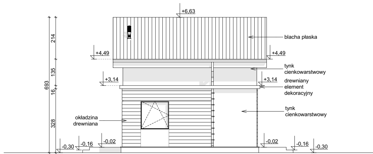
ELEWACJA BOCZNA
