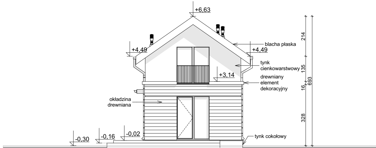
ELEWACJA OGRODOWA
