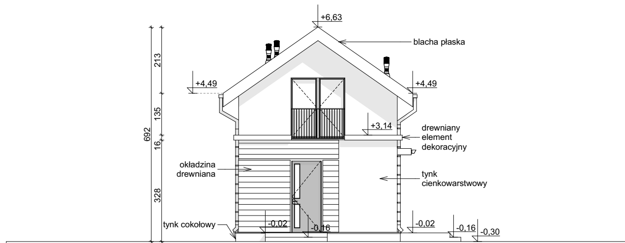
ELEWACJA FRONTOWA
