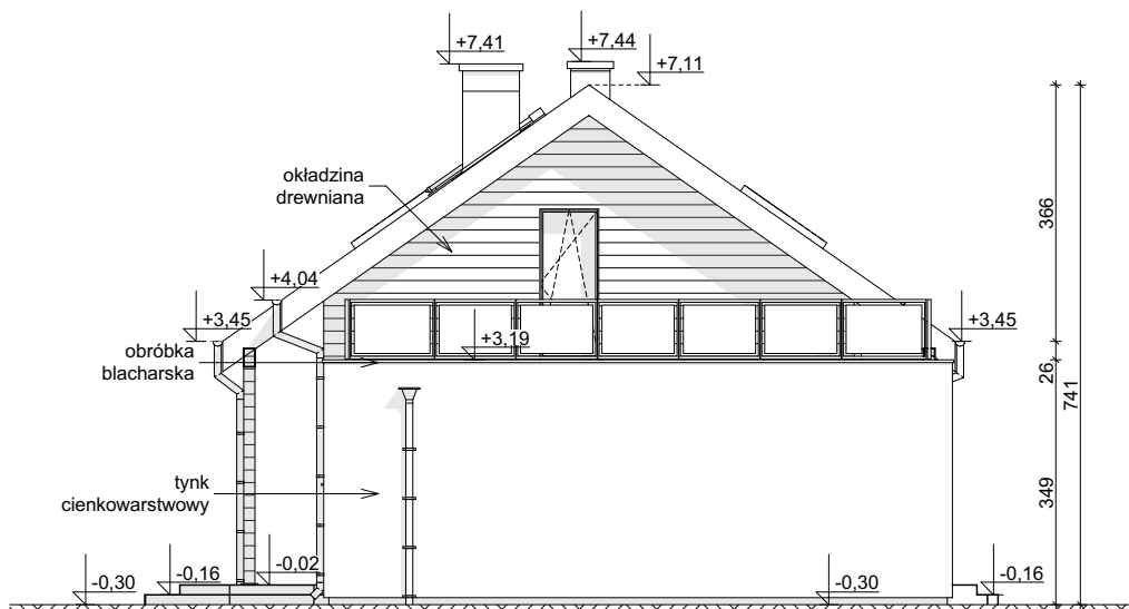
ELEWACJA BOCZNA
