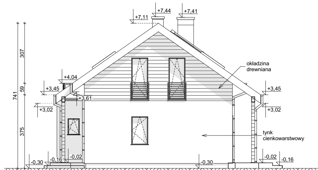
ELEWACJA BOCZNA
