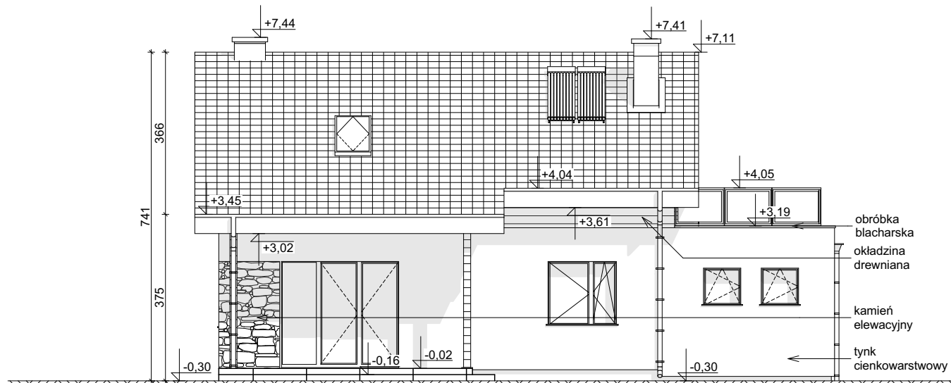
ELEWACJA OGRODOWA
