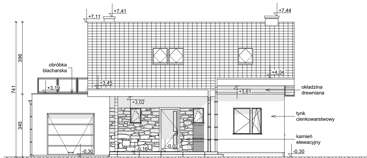
ELEWACJA FRONTOWA
