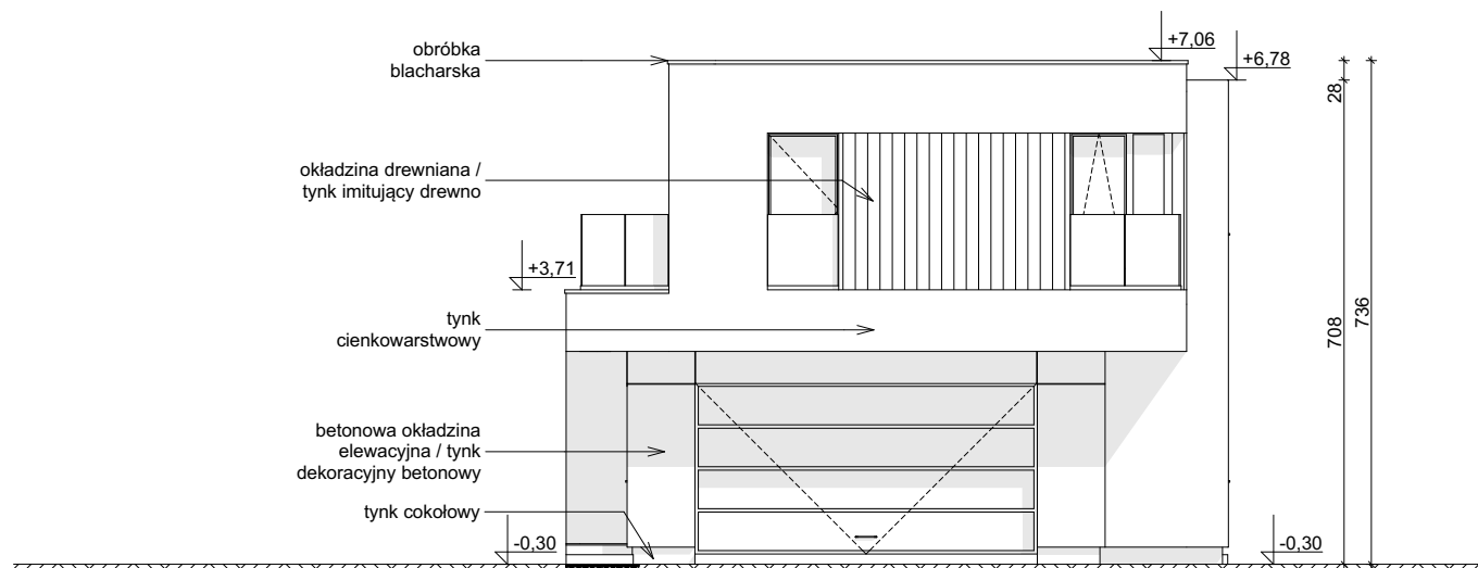
ELEWACJA BOCZNA
