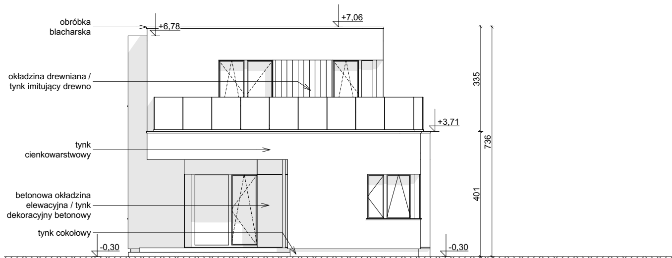
ELEWACJA BOCZNA
