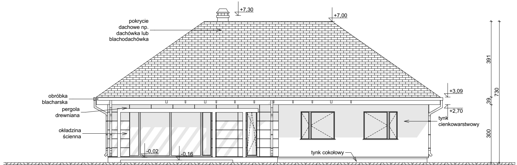
ELEWACJA OGRODOWA
