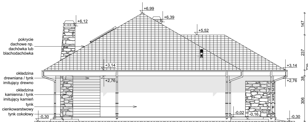
ELEWACJA BOCZNA
