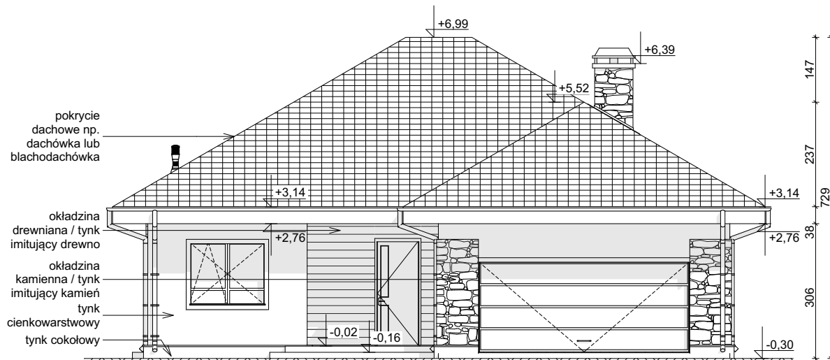
ELEWACJA FRONTOWA
