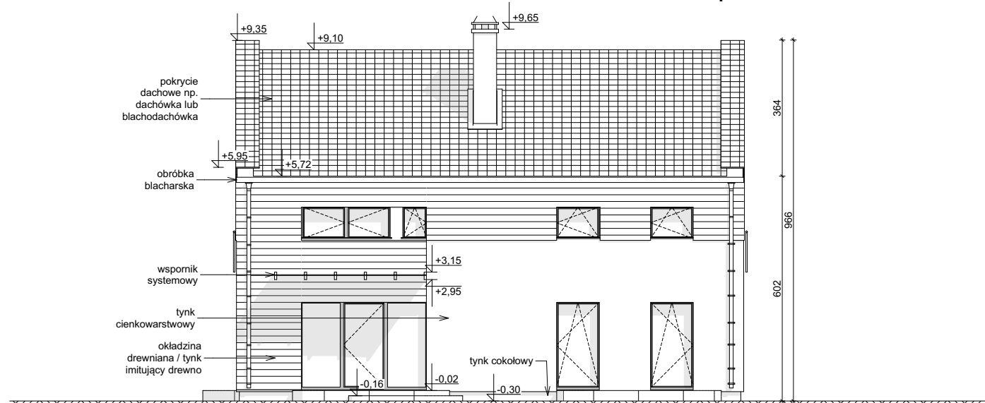
ELEWACJA OGRODOWA
