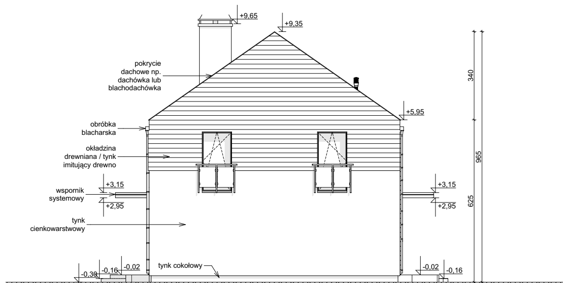
ELEWACJA BOCZNA
