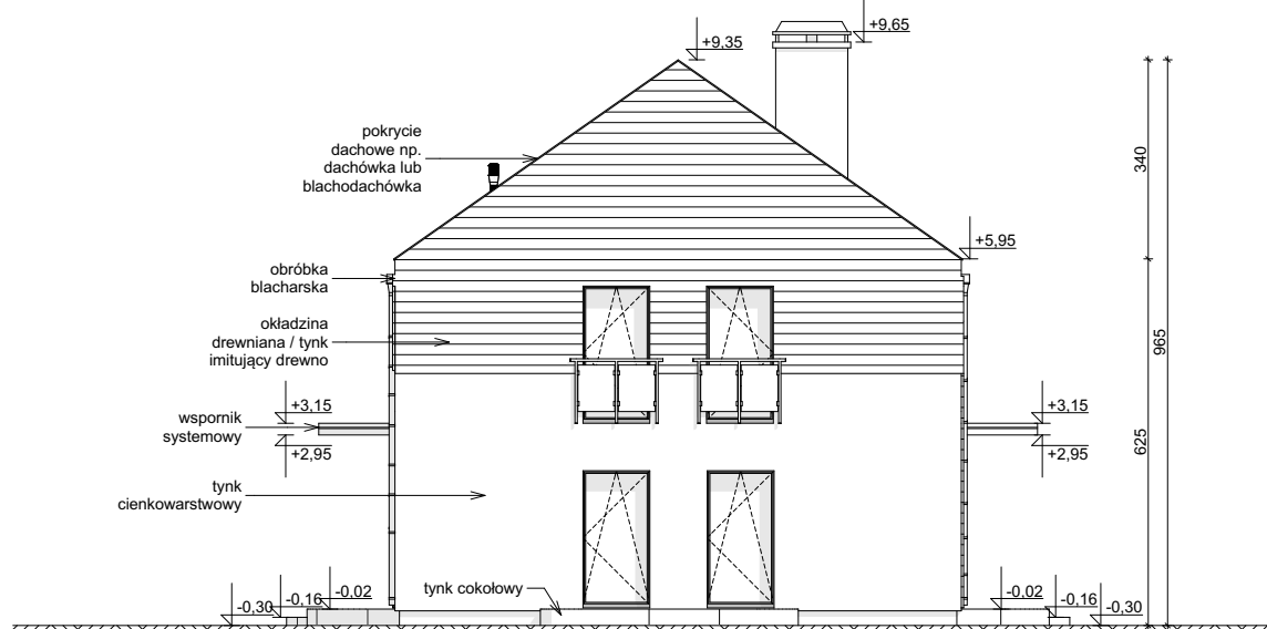
ELEWACJA BOCZNA
