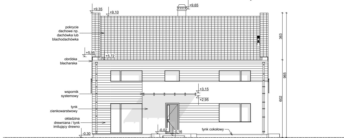
ELEWACJA FRONTOWA
