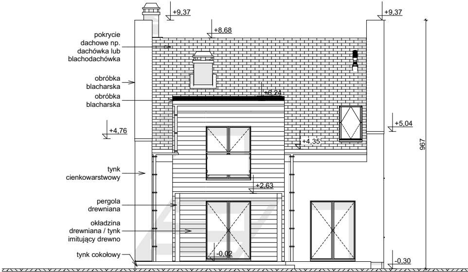
ELEWACJA OGRODOWA
