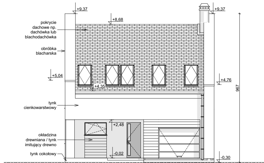
ELEWACJA FRONTOWA
