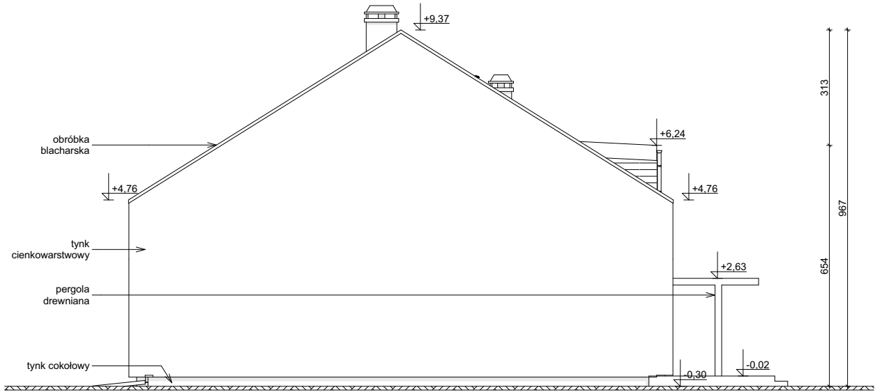
ELEWACJA BOCZNA
