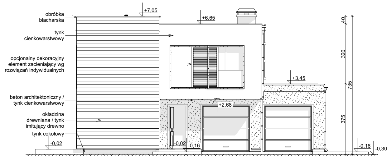
ELEWACJA FRONTOWA
