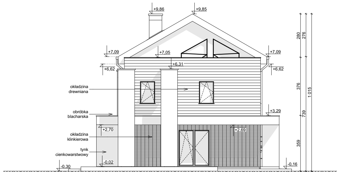
ELEWACJA BOCZNA
