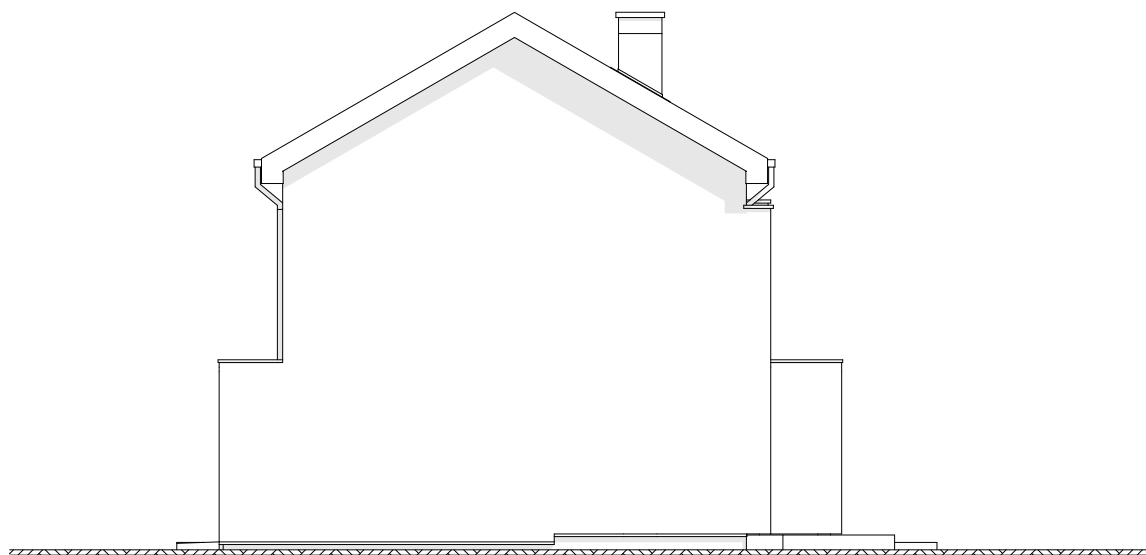
ELEWACJA BOCZNA
