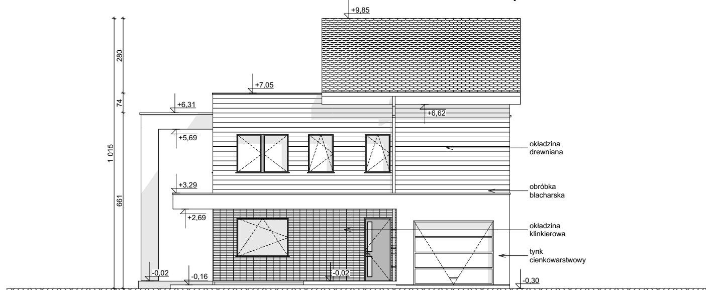
ELEWACJA FRONTOWA
