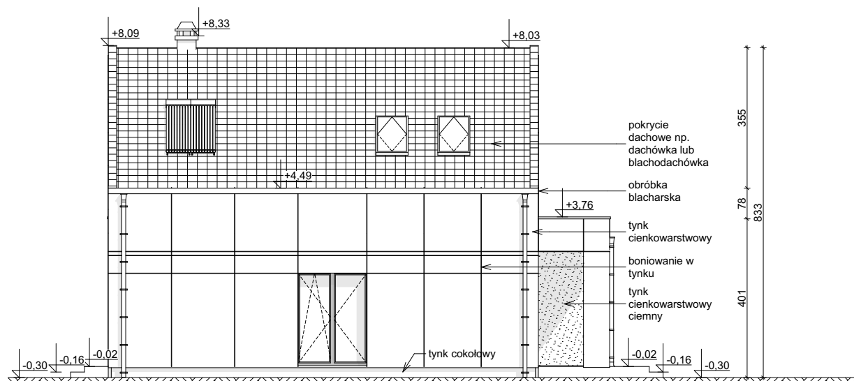
ELEWACJA BOCZNA
