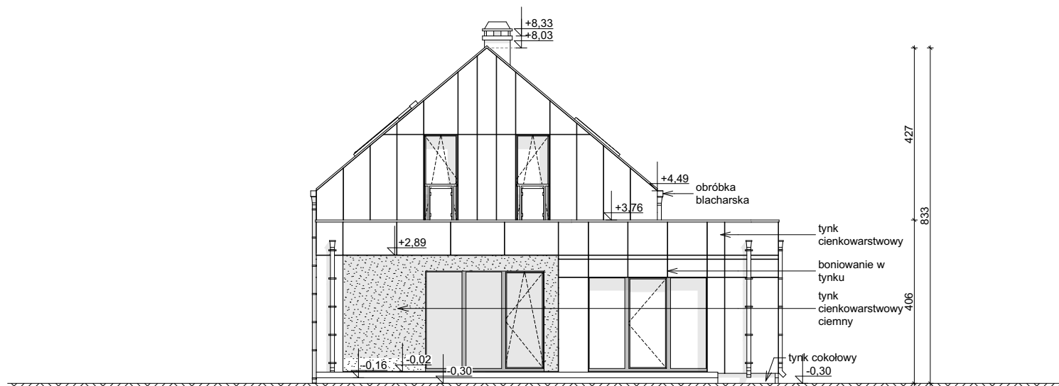
ELEWACJA OGRODOWA
