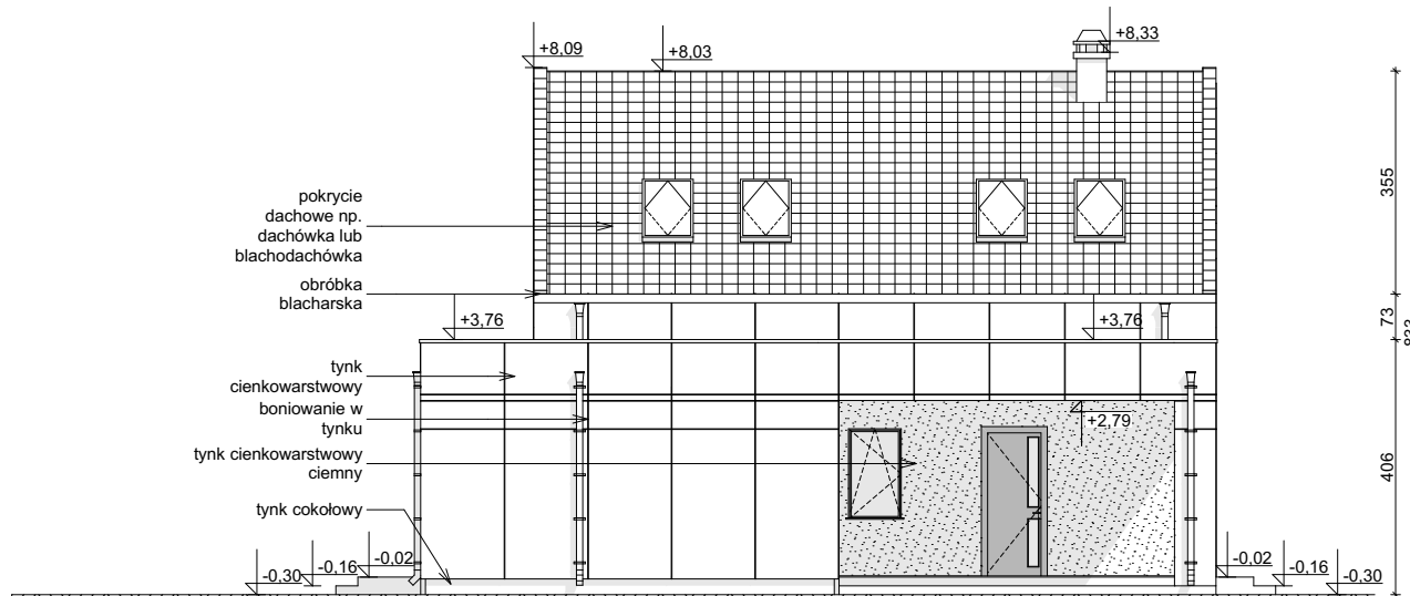
ELEWACJA BOCZNA
